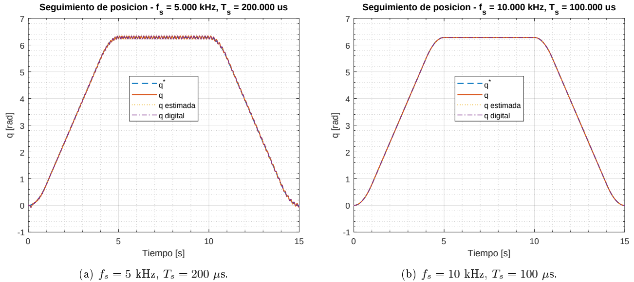
Figura 106: Detalle del efecto de la frecuencia de muestreo sobre la respuesta en posición.
