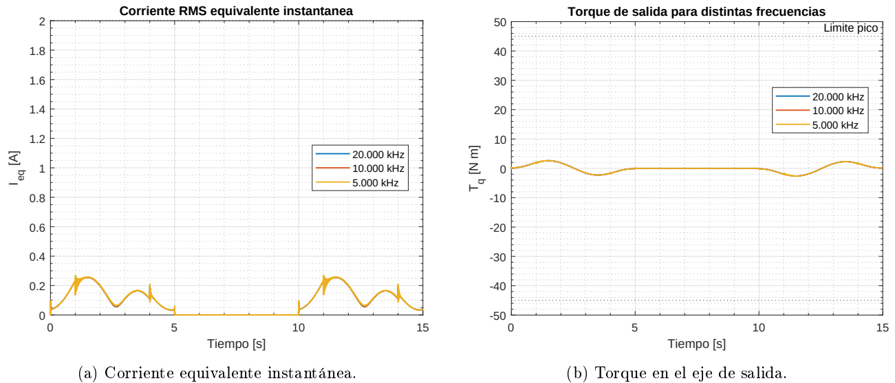
Figura 107: Esfuerzos de control para las frecuencias de muestreo evaluadas.
