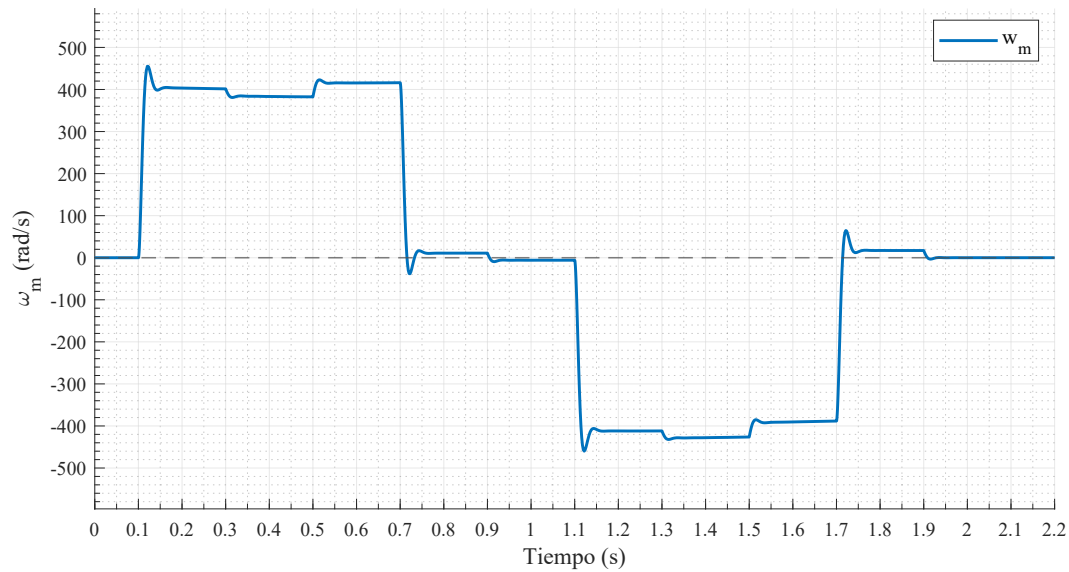
Figura 20: Evolución temporal de la velocidad angular del rotor \omega_m(t) .
