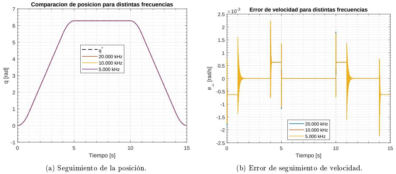
Figura 105: Comparación del desempeño para distintas frecuencias de muestreo.
