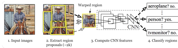
Figura 2.11. Esquema simplificado del funcionamiento de R-CNN, [37].
