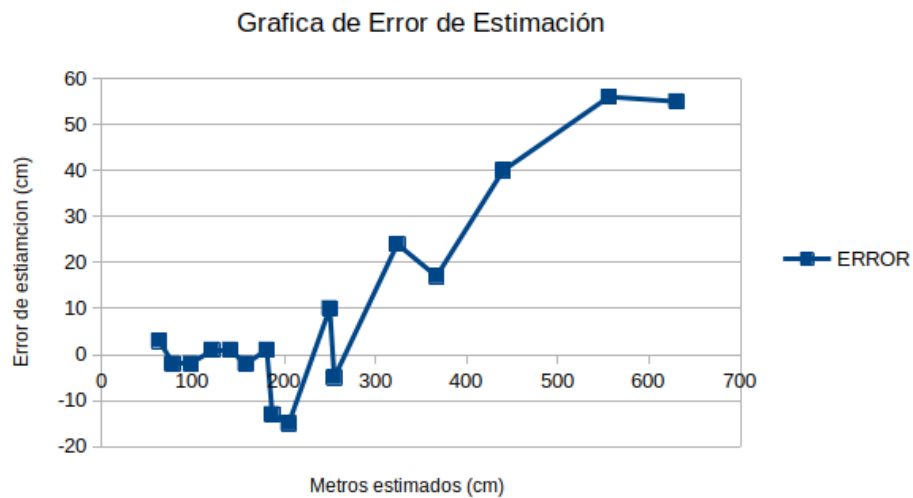
Figura 5.17: Error de estimación de distancia obtenido con la cámara real y el UAV objetivo real. (Imagen de Elaboración Propia)
