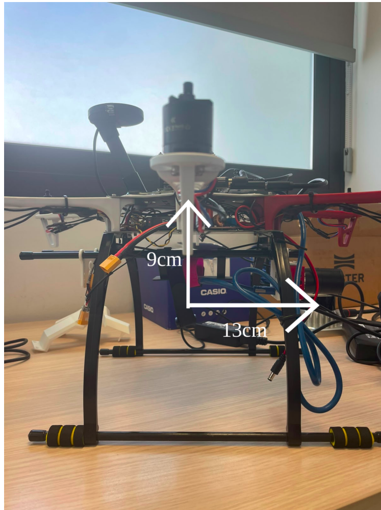
Figura 4.11. Montaje del dron cazador con la cámara utilizada en las pruebas reales. (Imagen de Elaboración Propia)
