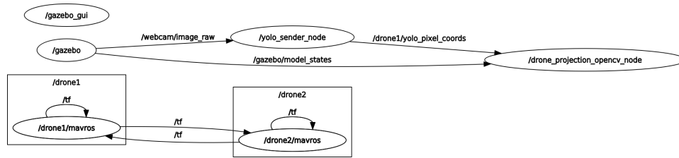
Figura 4.2. Grafo del sistema con los nodos de visión activados. Imagen de elaboración propia.
