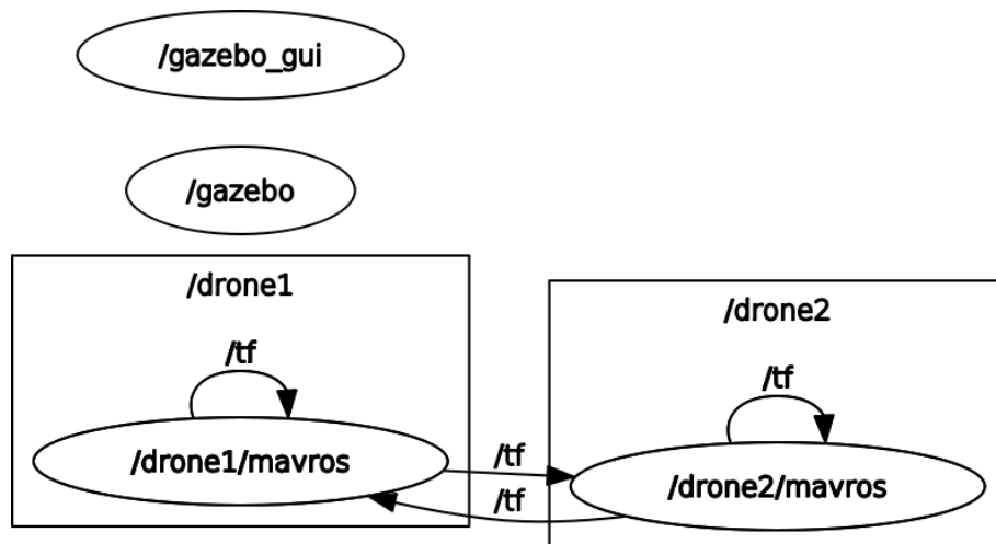
Figura 4.1. Grafo inicial del sistema sin nodos de visión ni control activos. Imagen de elaboración propia.
