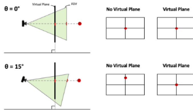
Figura 4.6. Esquema de compensación de actitud aplicado al plano de imagen.
