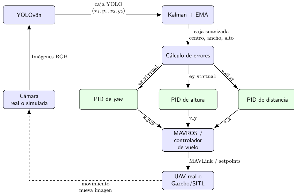
Figura 4.5: Arquitectura general del sistema de seguimiento visual, válida tanto para simulación como para despliegue real.
