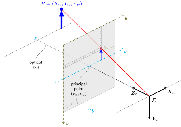
Figura 3.4. Esquema simplificado del modelo de cámara estenopeica. Fuente: [60].
