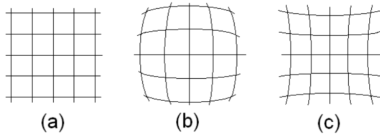
Figura 3.5. Imágenes de una pantalla de objeto rectangular mostradas con (a) ninguna distorsión; (b) distorsión radial; (c) distorsión tangencial., [67].
