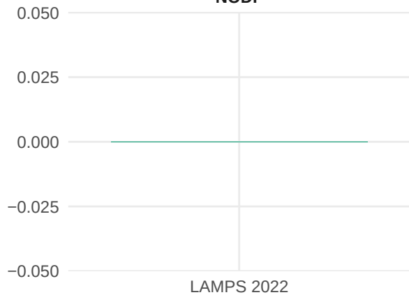
NODF
