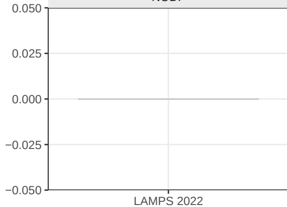
NODF
