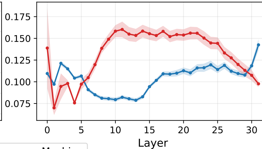
Anisotropy
