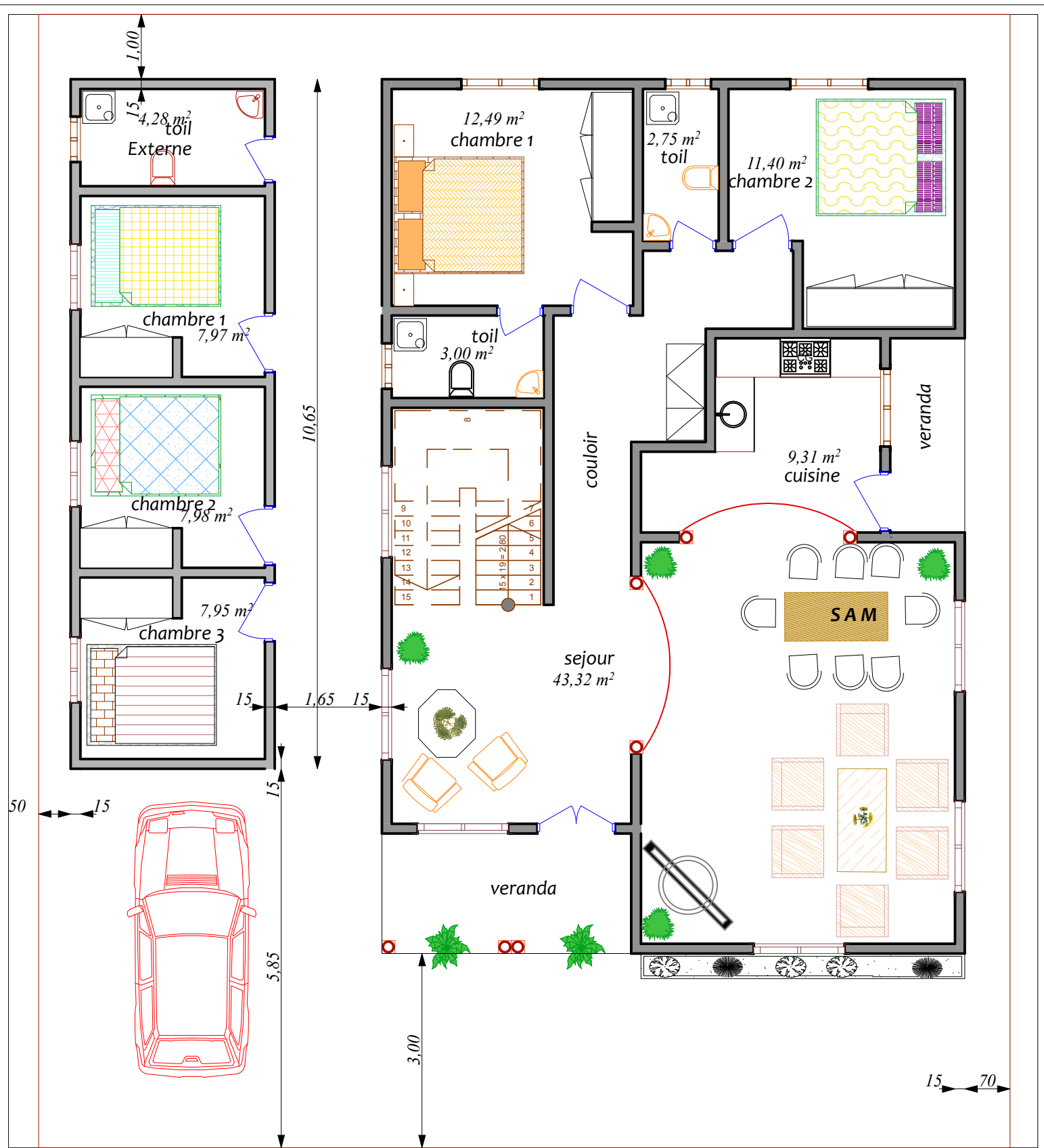
PROPOSITION AMENAGEMENT R D C EC 1:100
