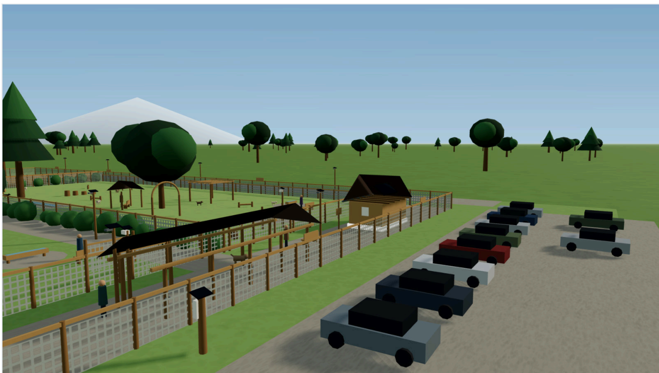
Figura D.2. Vista desde el estacionamiento. A la derecha, el baño público de dos recintos universales, en madera, con techo de fuerte pendiente, alero y paneles solares; a la izquierda, la zona de amarre techada de 12 x 3 m. Al fondo, el volcán Osorno.
