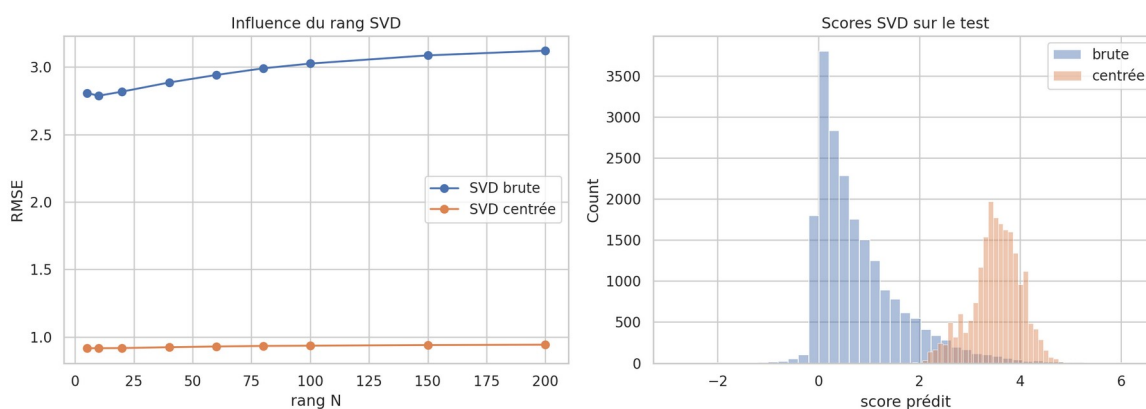
Figure 1 — Influence du rang et distribution des scores : SVD brute contre SVD centrée.
