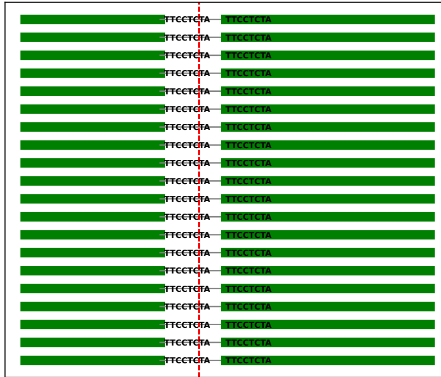
TK6 LIG4 -/- 4h
