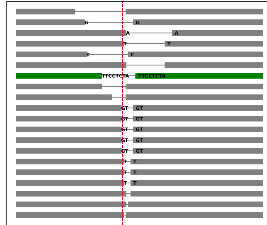
TK6 PolQ -/- 4h
