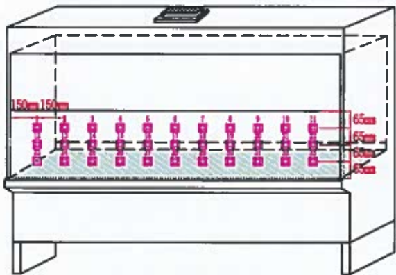
流入气流检测点位图
