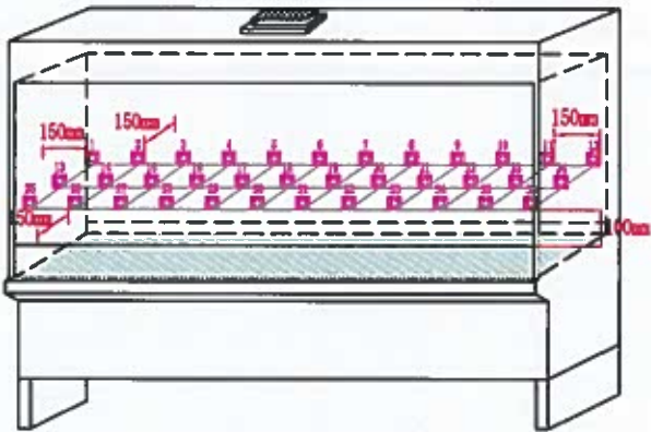
下降气流检测点位图
