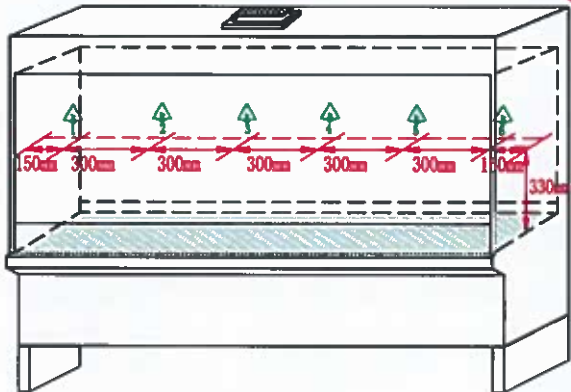
工作区照度检测点位图
