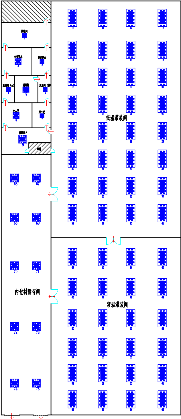
换气次数、静压差检测点位图
