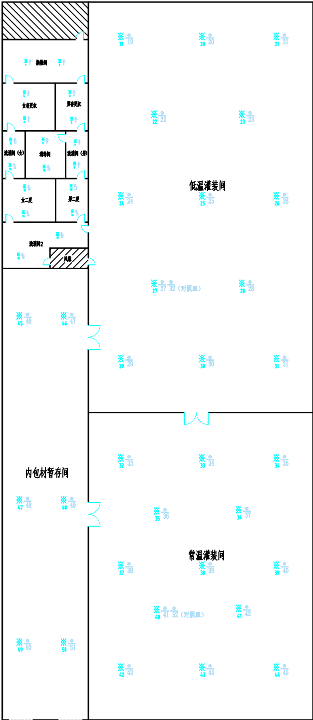
悬浮粒子数、沉降菌、浮游菌检测点位图
