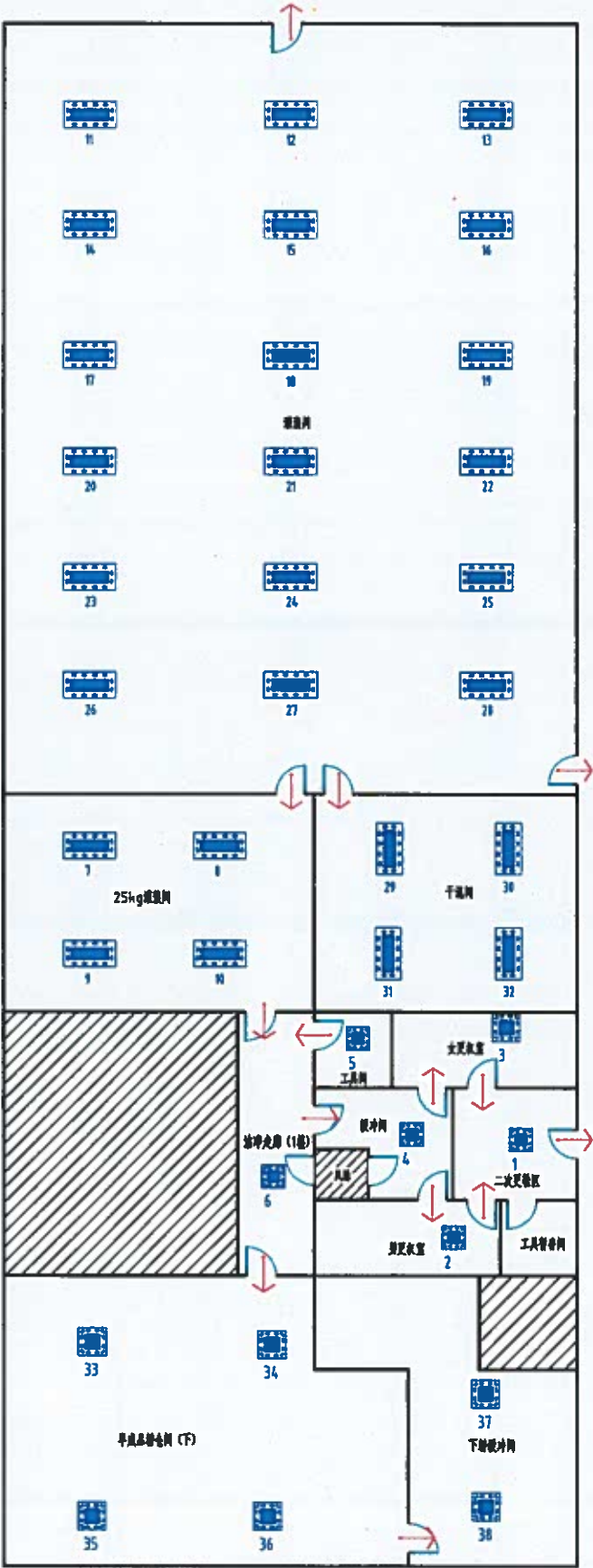
换气次数、静压差检测点位图
