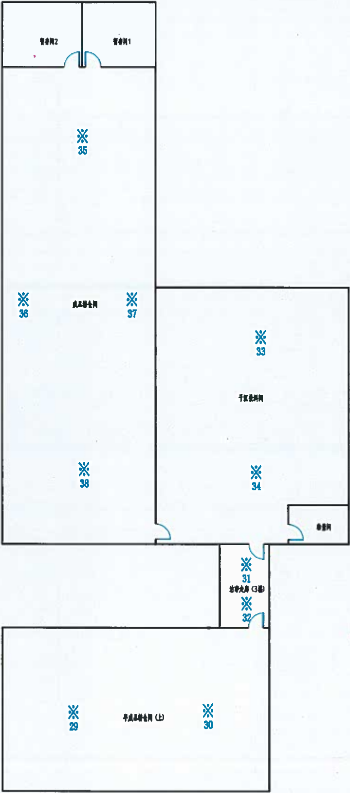
悬浮粒子数检测点位图
