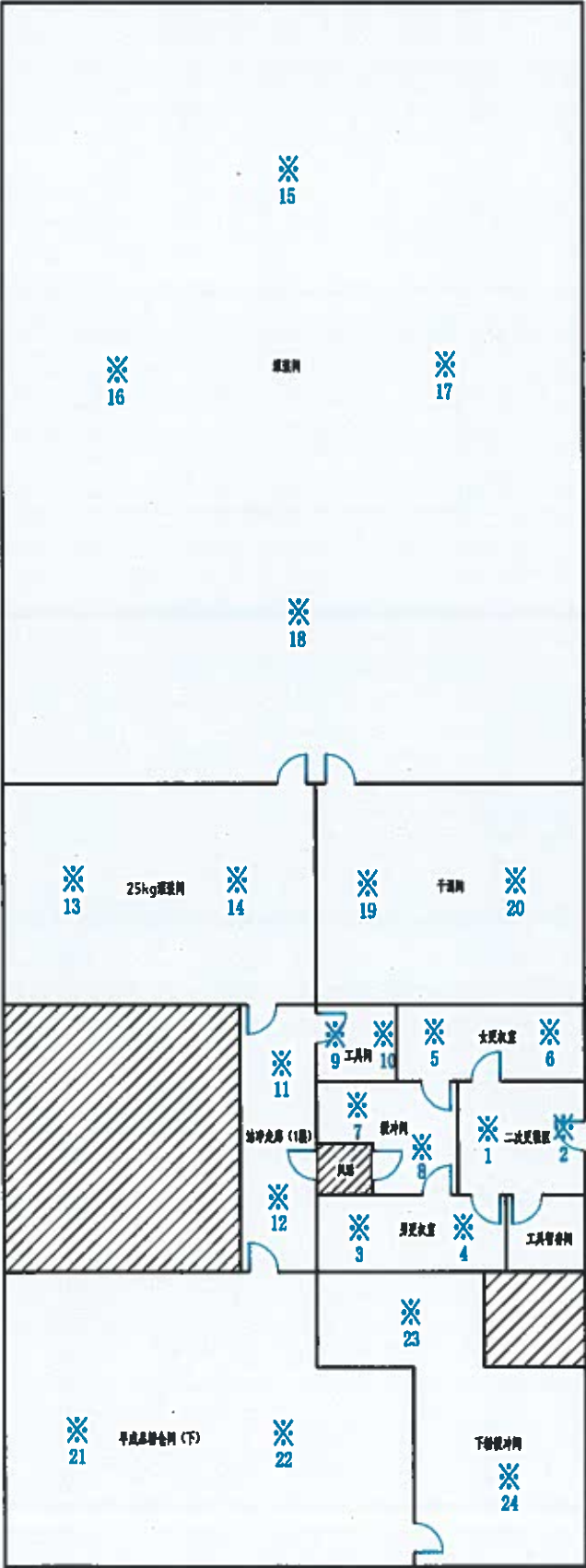
悬浮粒子数检测点位图
