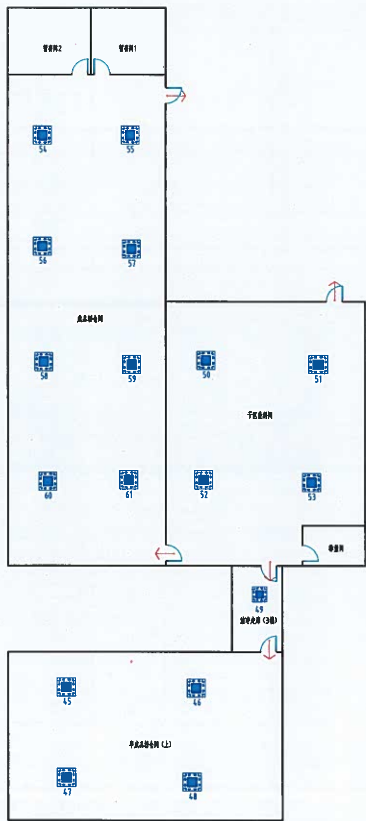
换气次数、静压差检测点位图
