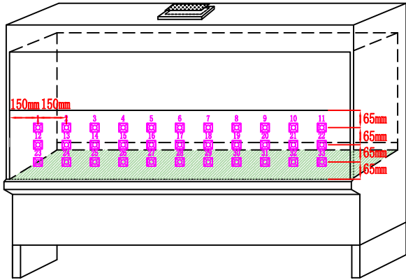
流入气流检测点位图
