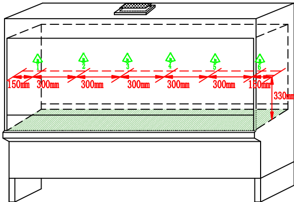
工作区照度检测点位图
