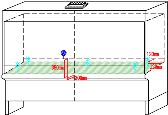
工作区悬浮粒子、噪声检测点位图
