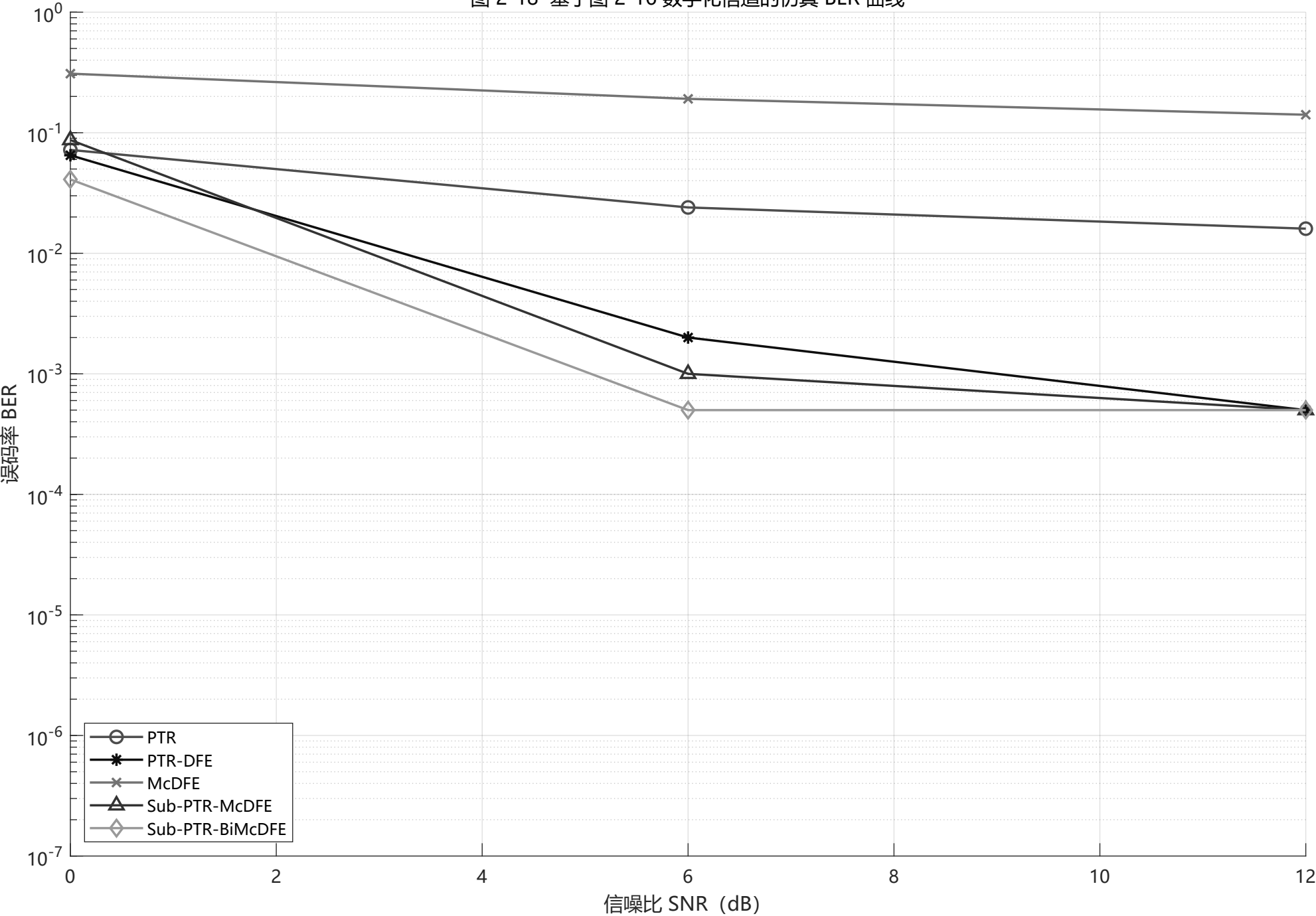
图 2-18 基于图 2-16 数字化信道的仿真 BER 曲线
