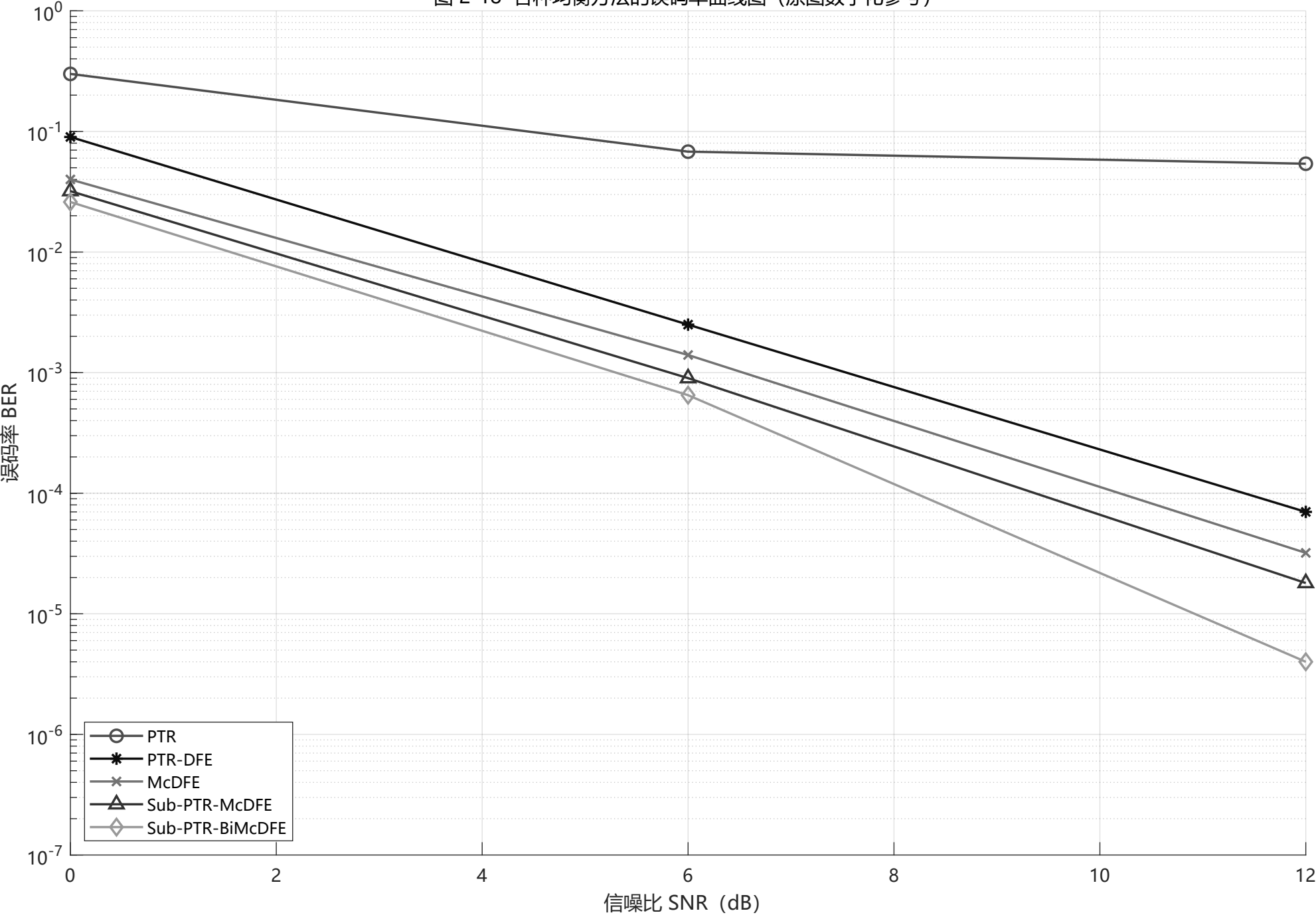
图 2-18 各种均衡方法的误码率曲线图 (原图数字化参考)
