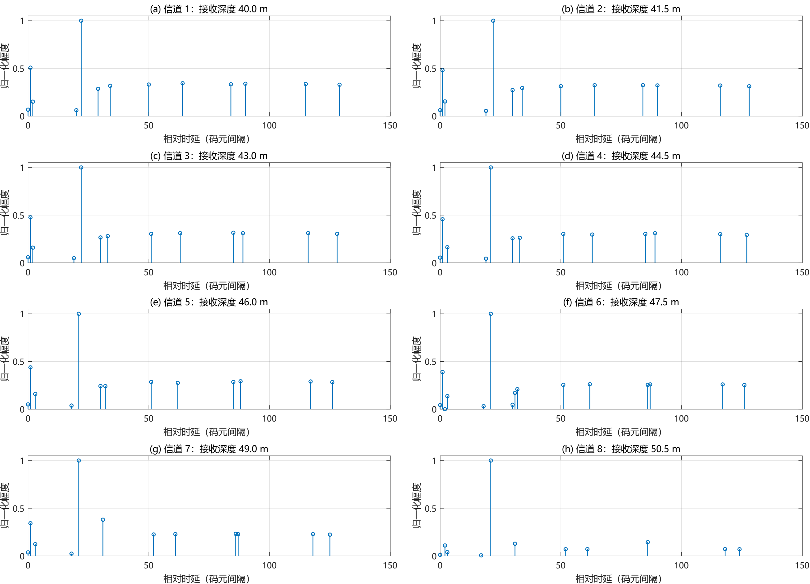
图 2-16 Bellhop 仿真得到的八阵元多径信道
