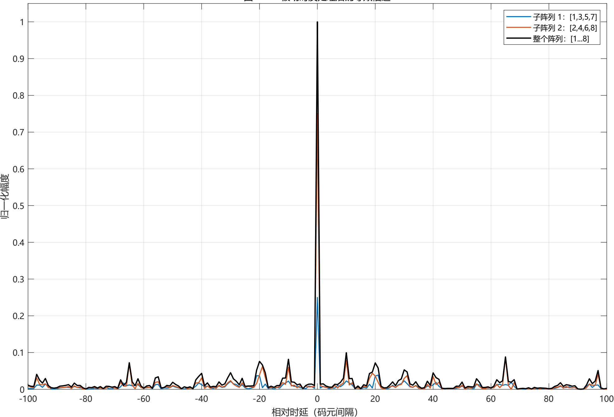
图 2-17 被动时反处理后的等效信道
