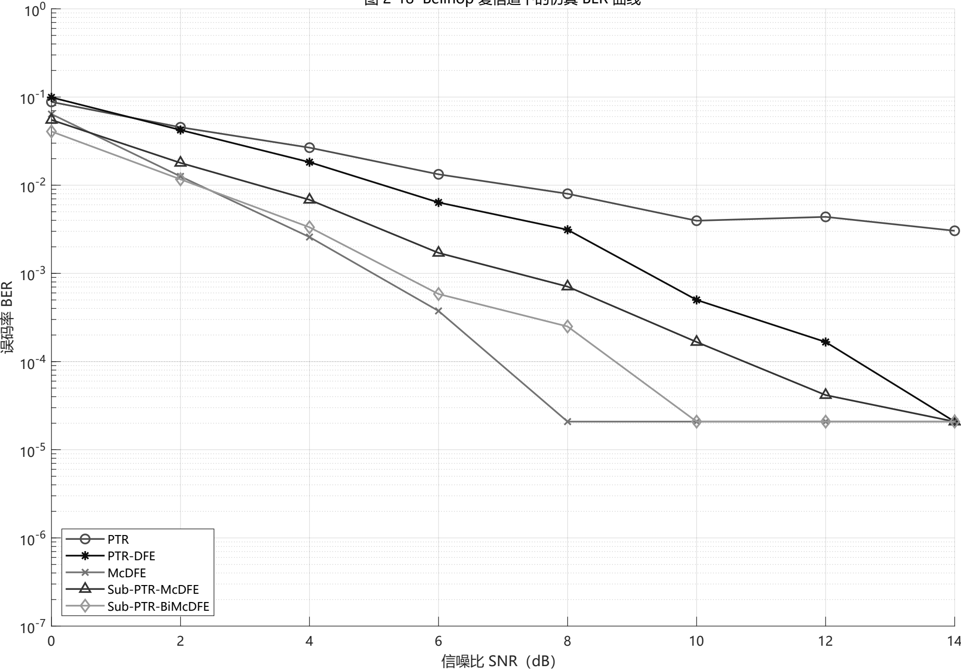
图 2-18 Bellhop 复信道下的仿真 BER 曲线
