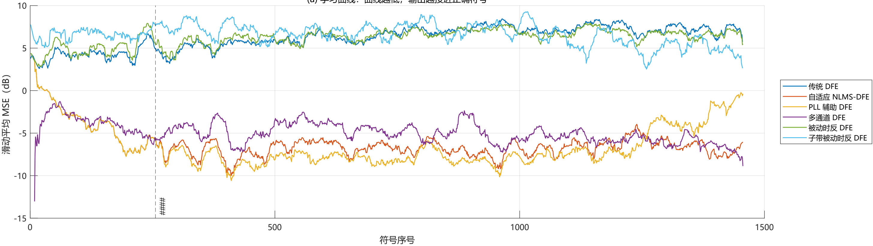
(b) 自适应 NLMS-DFE：判决前连续输出
