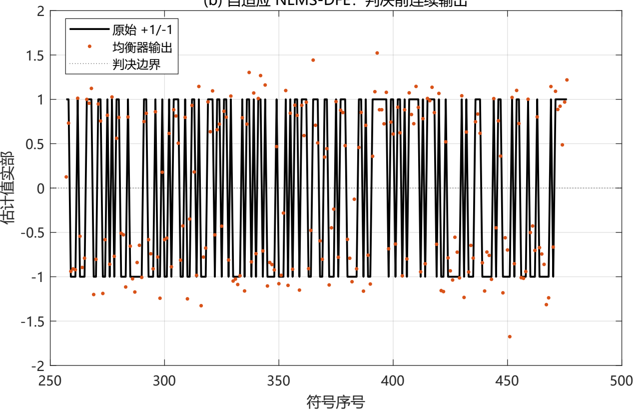
(b) 自适应 NLMS-DFE：判决前连续输出
