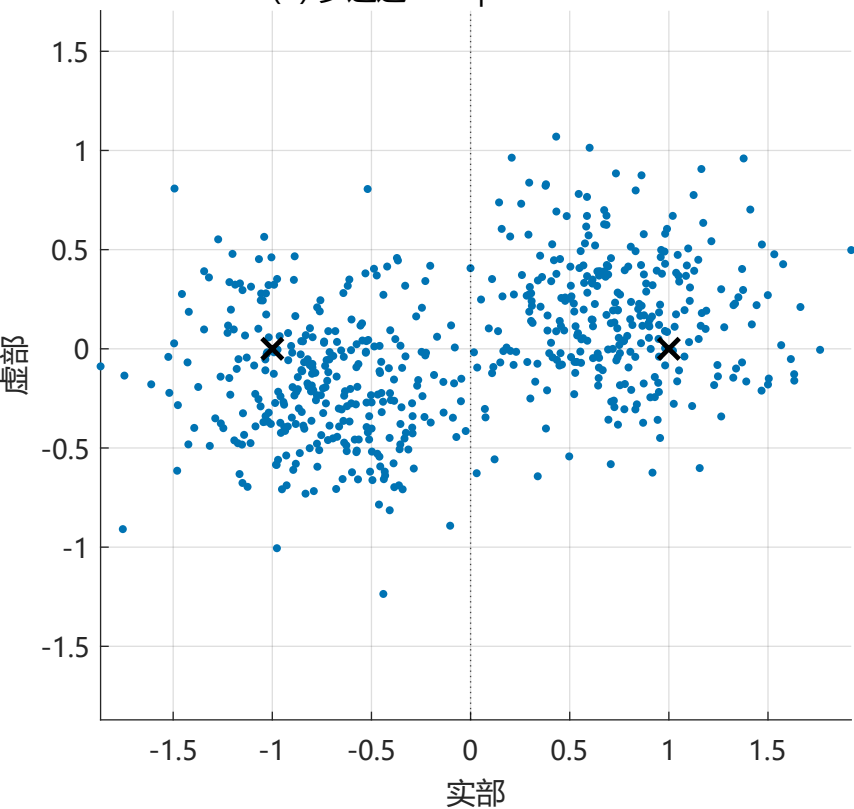
(d) 多通道 DFE | BER = 0.0275
