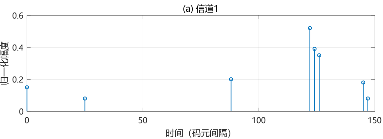
图 2-16 按原图数字化的八阵元多径信道
