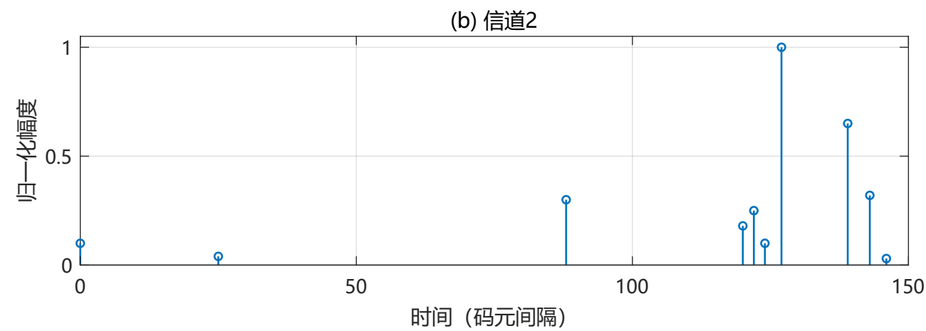
图 2-16 按原图数字化的八阵元多径信道
