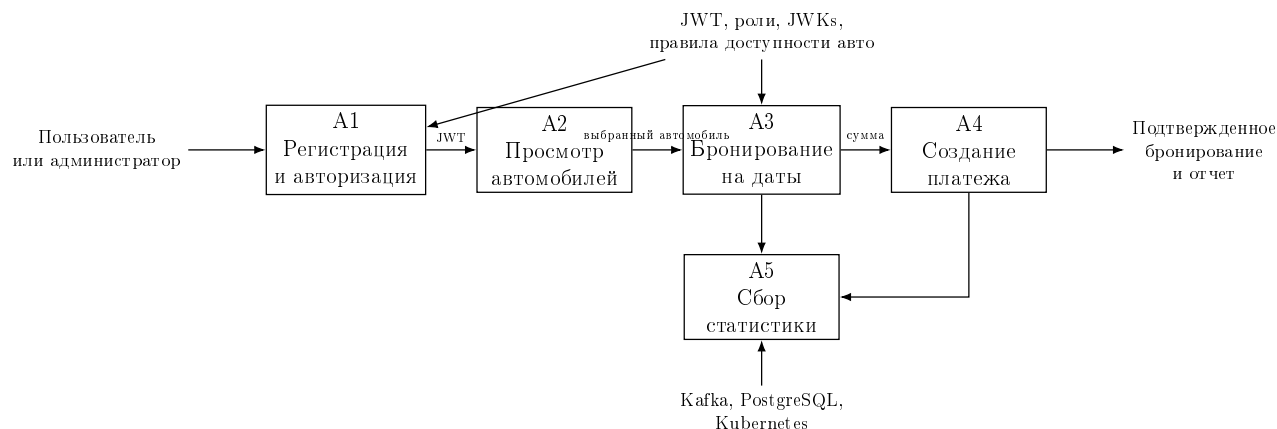
Рисунок 2.2 – Детализированная концептуальная модель системы в нотации IDEF0
