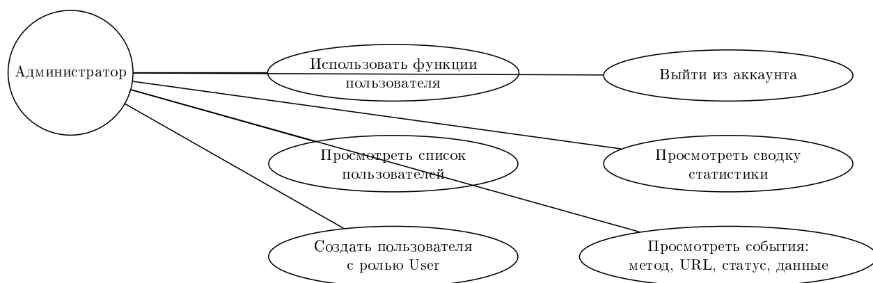
Рисунок 2.5 – Диаграмма прецедентов с точки зрения администратора
