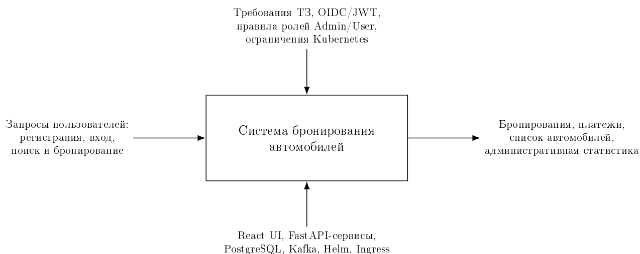
Рисунок 2.1 – Концептуальная модель системы в нотации IDEF0
