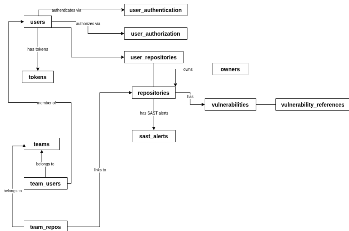
Figura 4.1: diagrama do modelo de dados
