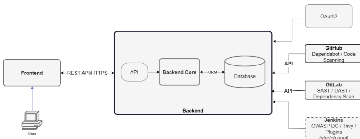
Figura 3.1: diagrama da arquitetura
