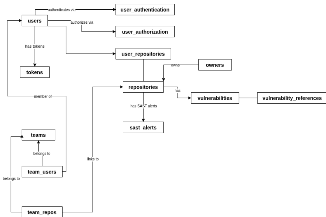
Figura 3.2: Diagrama do modelo de dados ilustrando sucintamente as ligações entre cada uma das entidades que o constituem
