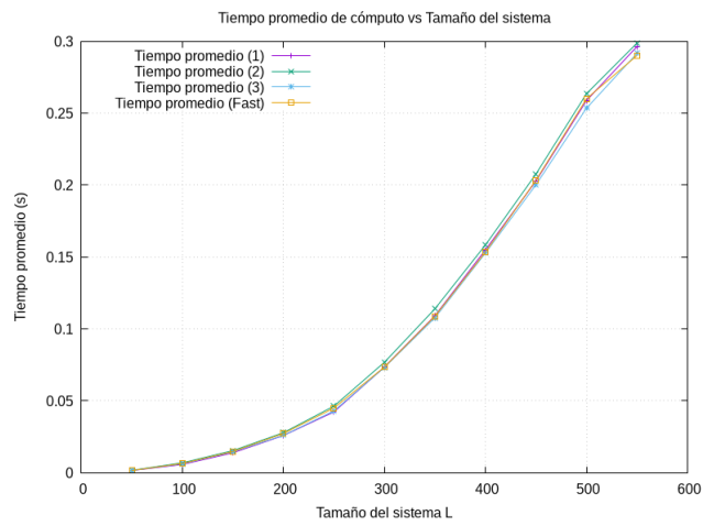
Figure 1: Grafica del tiempo de computo (CPU) en funcion del tamaño del sistema L .
