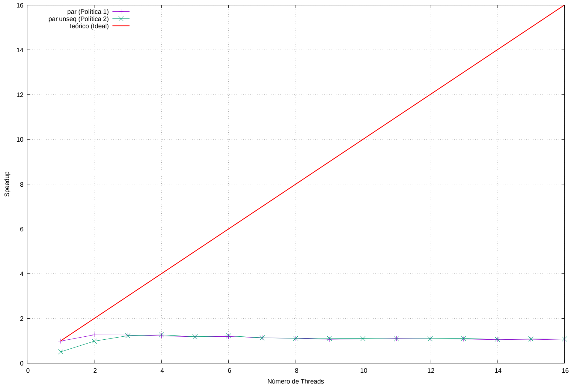
Speedup - Vector Size: 2e8 - Cores Físicos: 8, Hilos Totales: 16
