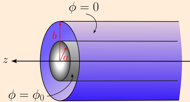
Figura 3.8: Cilindros coaxiales.
