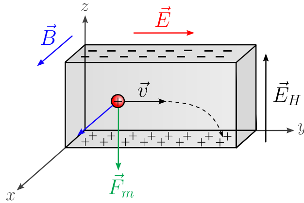
Figura 5.6: Efecto Hall.
