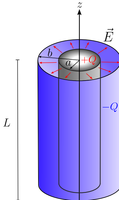
Figura 3.17: Capacitador cilíndrico.
