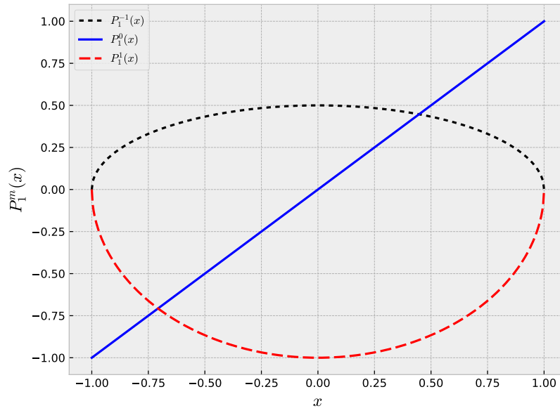
Figura 5.5: Funciones Asociadas de Legendre: n = 1 .
