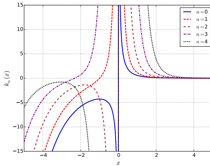
Figura 6.10: Primeras cinco funciones esféricas modificadas de Bessel de segunda especie (funciones de Neumann) de orden entero. Código Python aquí .
