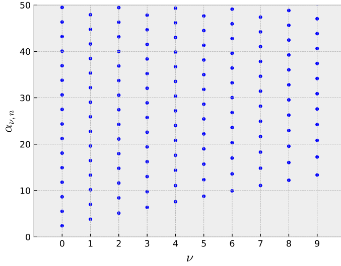
Figura 6.1: Algunos ceros de las funciones J_\nu(x) de orden entero. Código Python disponible en este notebook.
