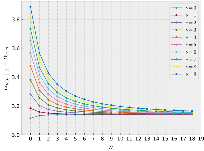
Figura 6.2: Diferencias entre ceros sucesivos de las funciones J_\nu(x) de orden entero. Código Python disponible en este notebook.
