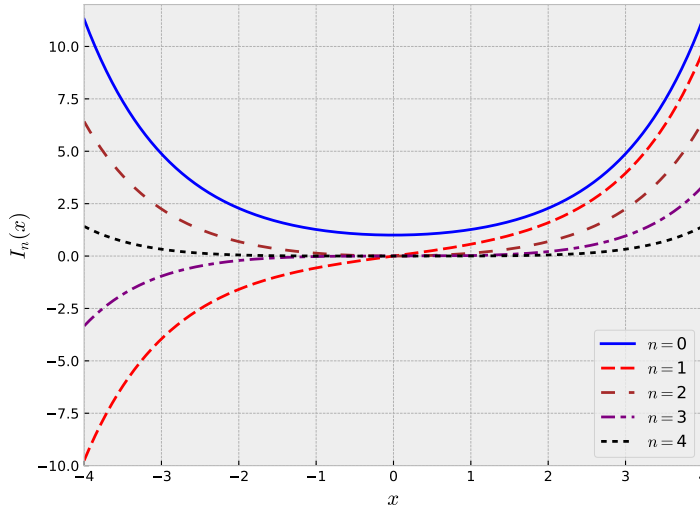
Figura 6.5: Primeras cinco funciones modificadas de Bessel (de primera especie) de orden entero. Código Python aquí .
