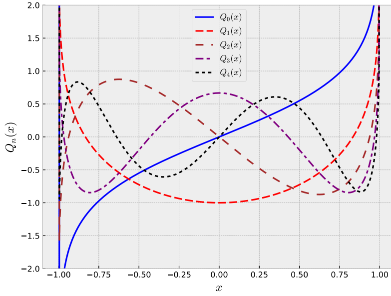
Figura 5.4: Primeras cinco funciones de Legendre de segunda especie.
