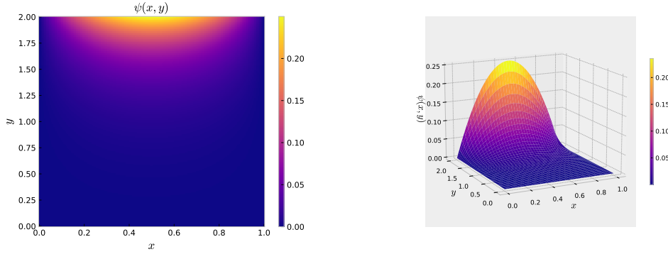
Figura 4.1: La solución a nuestro problema, en 3D y colores. Código Python aquí .
