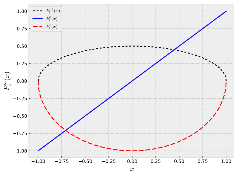
Figura 5.5: Funciones Asociadas de Legendre: n = 1 .
