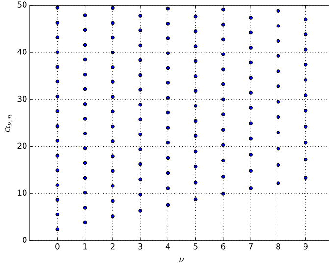
Figura 6.1: Algunos ceros de las funciones J_\nu(x) de orden entero. Código Python disponible en este notebook.
