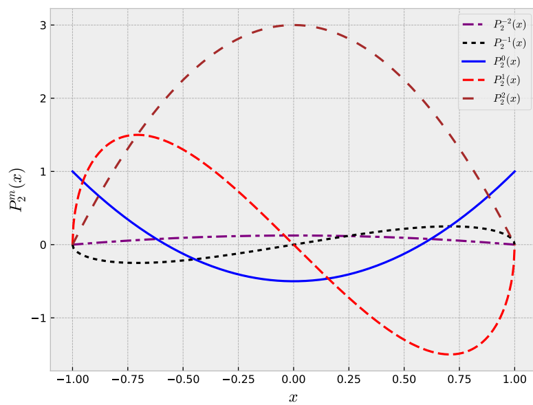
Figura 5.6: Funciones Asociadas de Legendre: n = 2 .
