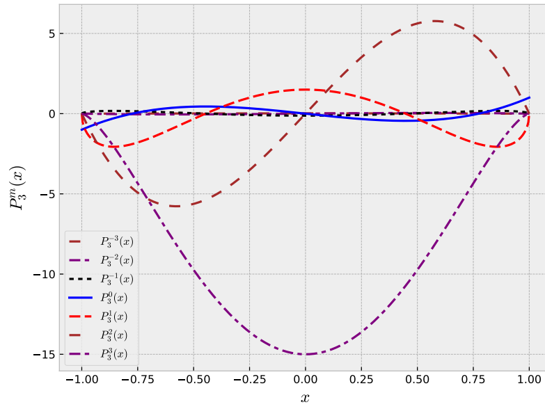
Figura 5.7: Funciones Asociadas de Legendre: n = 3 .
