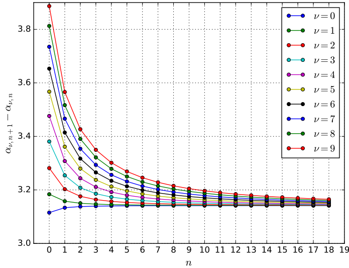
Figura 6.2: Diferencias entre ceros sucesivos de las funciones J_\nu(x) de orden entero. Código Python disponible en este notebook.
