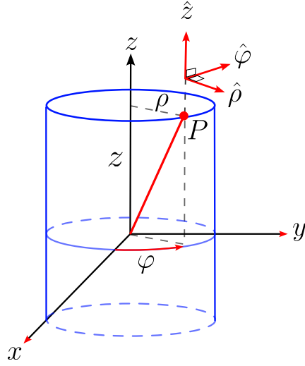
Figura B.1: Coordenadas cilíndricas (\rho, \varphi, z) y sus vectores unitarios.
