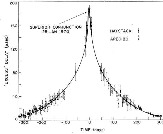
Figura 3.4: Mediciones de Radar del efecto Shapiro [37].
