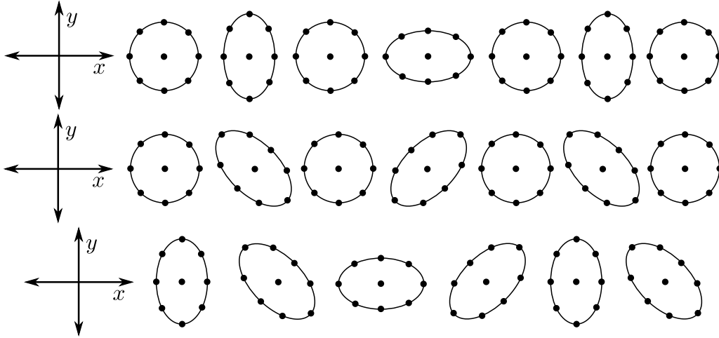
Figura 6.1: Oscilaciones inducidas por una onda gravitacional con polarización +, \times y circular. Figuras adaptadas a partir de originales en [21].
