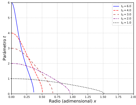
Figura 10.1: Solución de ec. TOV: t v/s x .
