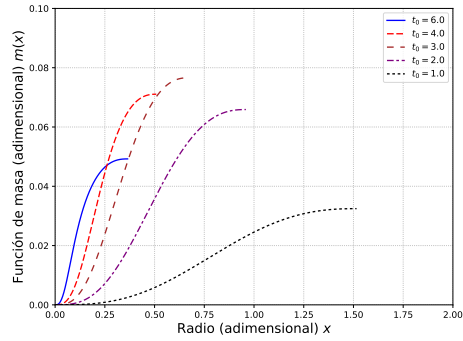
Figura 10.2: Solución de ec. TOV: m v/s x .
