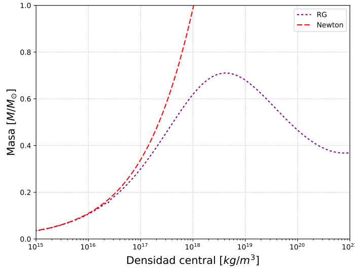
Figura 10.3: Relación masa-densidad central para estrellas de neutrones con las ecuaciones TOV y newtonianas
