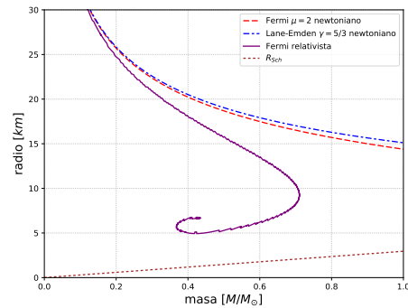
Figura 10.5: Relación Masa-Radio para estrellas de neutrones con las ecuaciones TOV y newtonianas
