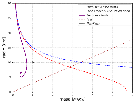
Figura 10.4: Relación Masa-Radio para estrellas de neutrones con las ecuaciones TOV y newtonianas
