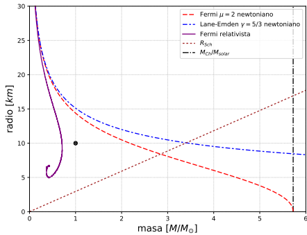
Figura 10.4: Relación Masa-Radius para estrellas de neutrones con las ecuaciones TOV y newtonianas
