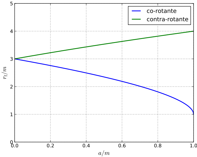
Figura 5.8: Radios mínimos para órbitas circulares ecuatoriales.
