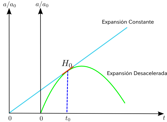
Figura 7.5: Como se puede observar del gráfico, si la expansión es desacelerada el tiempo transcurrido desde a = 0 hasta a_0 es menor que el de un modelo de expansión a velocidad constante.
