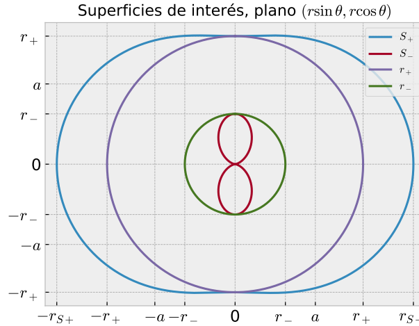
Figura 5.2: Horizontes y superficies de redshift infinito de la solución de Kerr. Código Python aquí .
