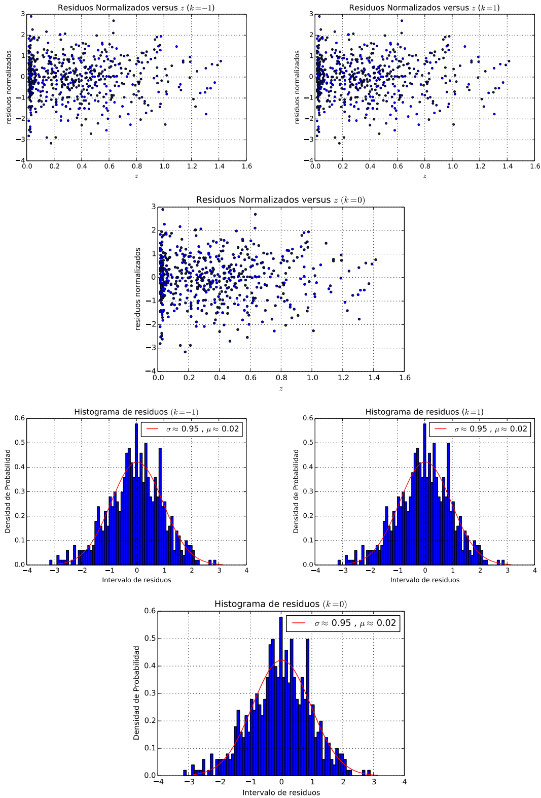
Figura 7.10: Diagrama de residuos correspondientes a los tres distintos valores de k , con sus respectivos histogramas.
