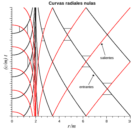
Figura 4.1: Curvas nulas radiales en coordenadas de curvatura.
