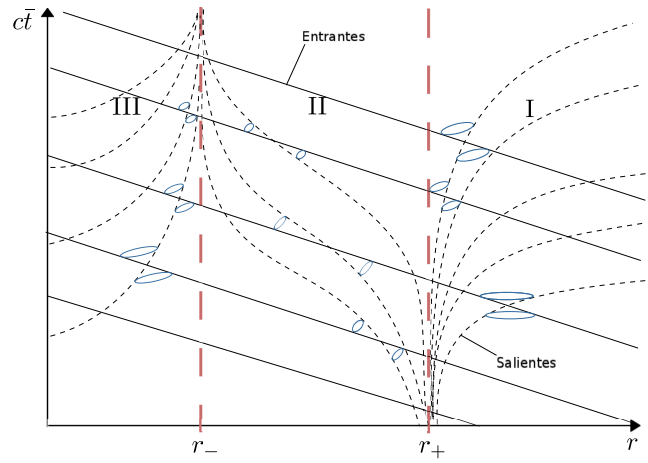
Figura 5.6: Diagrama de espacio tiempo en coordenadas de Eddington-Finkelstein.
