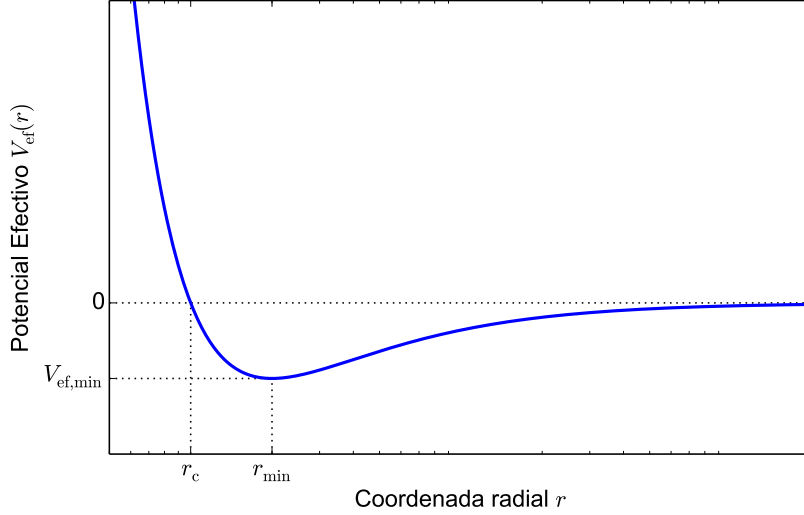
Figura A.1: Potencial newtoniano efectivo. Coordenada radial graficada en escala logarítmica.
