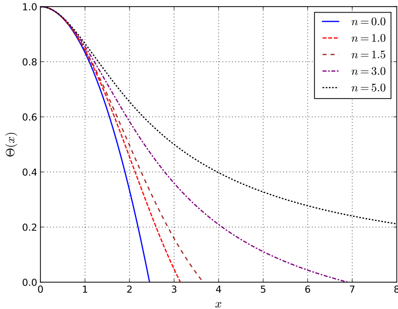
Figura 9.1: Algunas soluciones de la ecuación de Lane-Emden, con n = 1/(\gamma - 1) . Código Python aquí (G. Neumann).
