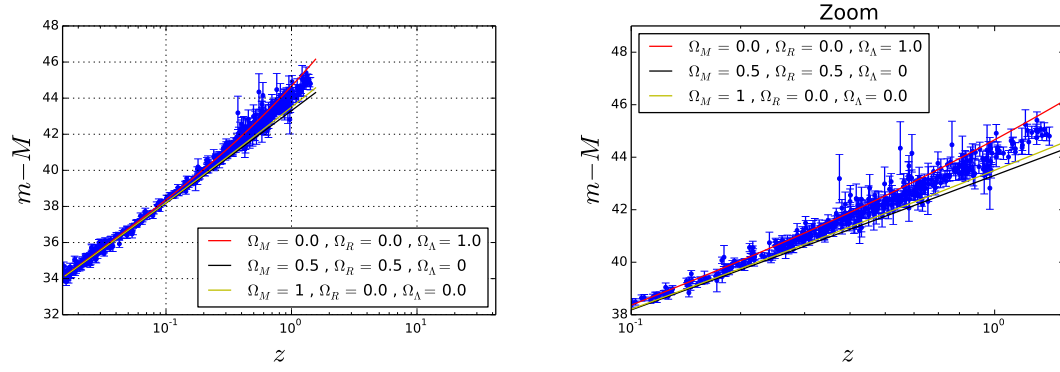
Figura 7.11: El gráfico de la izquierda corresponde a las curvas del modelo con k = 0 , para algunos valores de los parámetros asignados por nosotros. El gráfico de la derecha corresponde a un zoom de la parte superior del gráfico de la izquierda. Las tres curvas para redshifts pequeños se ajustan bien los datos, pero para redshifts mayores toma mayor importancia el tipo de materia presente en el universo.
