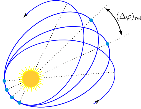
Figura 3.2: Corrimiento del perihelio (adaptada a partir de esta figura original).
