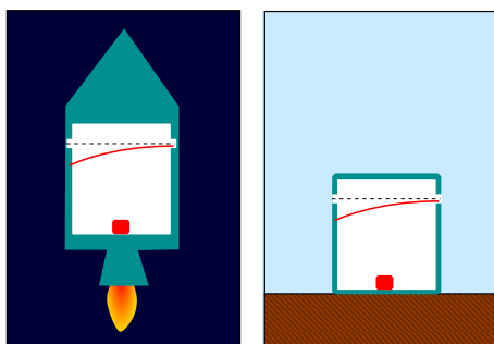
Figura 1.6: Deflexión de la luz. Ambos SR's aceleran respecto a SRLI's.
