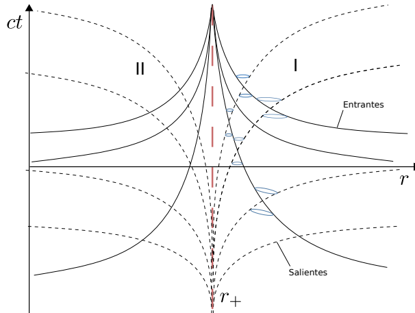
Figura 5.5: Diagrama espacio-tiempo en la vecindad de r_+
