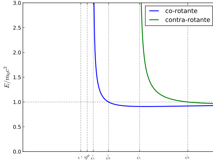
Figura 5.9: Energías de órbitas circulares ecuatoriales, para a = 0.6m . Código Python aquí .
