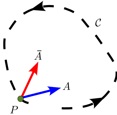
Figura 2.7: Transporte paralelo de un vector sobre una curva cerrada.
