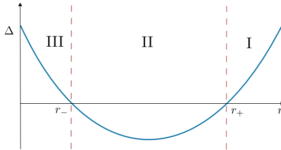
Figura 5.4: Función \Delta versus coordenada r
