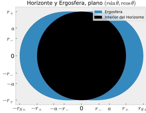
Figura 5.3: Horizonte de eventos y Ergosfera de la solución de Kerr. Código Python aquí .
