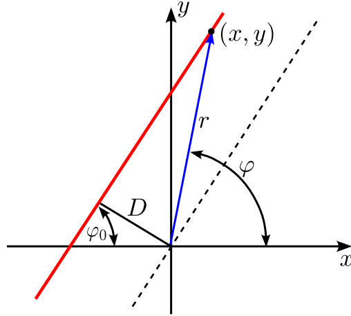
Figura 3.3: Solución newtoniana para el movimiento del rayo de luz.
