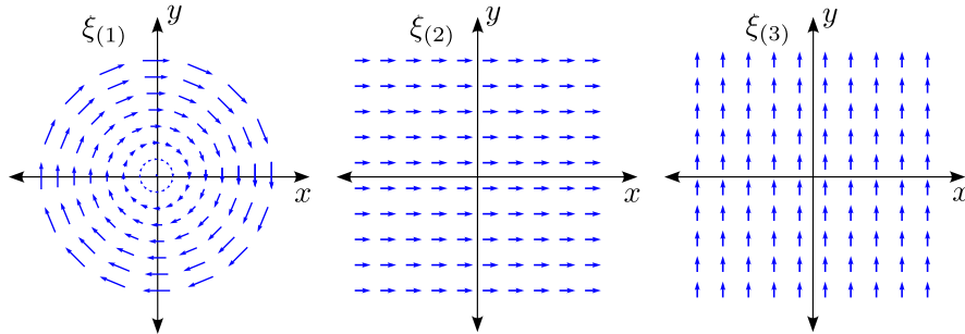
Figura 2.5: Vectores de Killing en el plano euclideo bidimensional.
