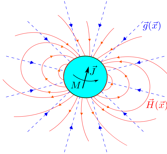
Figura 8.2: Líneas de campo gravitoelectrónico y gravitomagnético, producidas por una distribución esféricamente simétrica de masa total M y que rota con momentum angular total constante \vec{J} .
