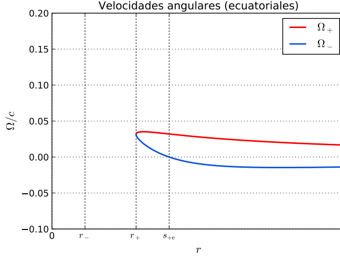
Figura 5.7: Frecuencias angulares permitidas para órbitas circulares ecuatoriales. Código Python aquí .
