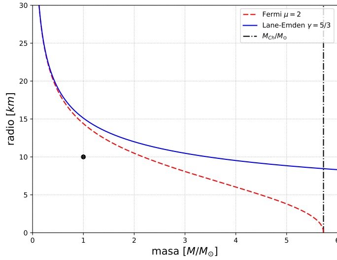
Figura 9.5: Relación masa-radio para estrellas de neutrones compuestas un gas de neutrones completamente degenerado en los casos límite no relativista ( \gamma = 5/3 ) y ultra relativista ( \gamma = 4/3 ). Se destaca, además, el valor más nombrado en la literatura para la masa y el radio de estas estrellas ( 1 M_{\odot} , 10[km] ).
