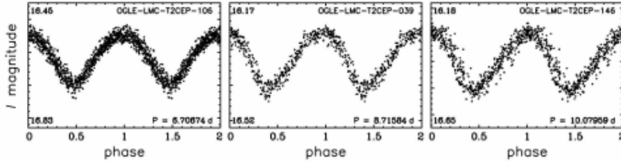
Figura 7.3: Curvas de luz de tres Cefeidas ordinarias tipo II, con periodos similares [?].
