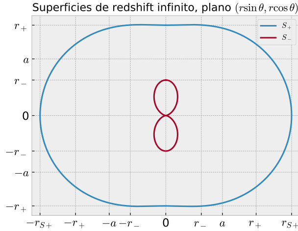
Figura 5.1: Superficies de redshift infinito. Código Python aquí .
