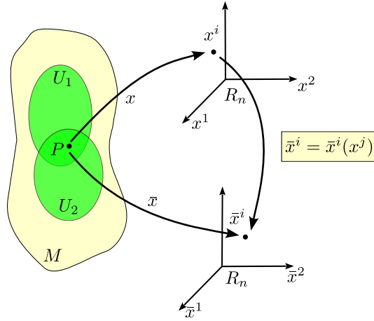
Figura 2.2: Una variedad y dos sistemas coordenados.
