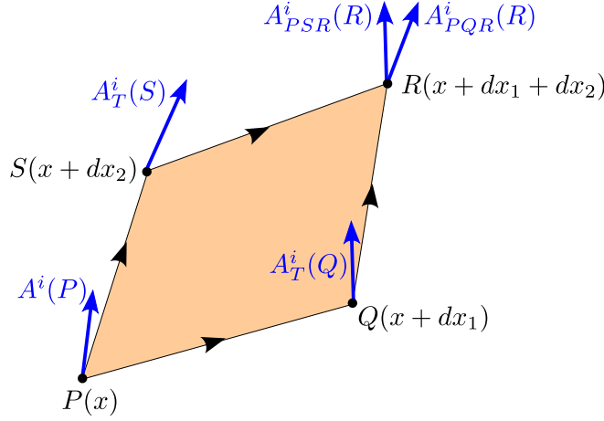
Figura 2.8: Transporte de un vector desde P a R por dos trayectorias (infinitesimales) distintas.
