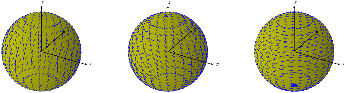
Figura 2.6: Vectores de Killing sobre la esfera: \xi_{(1)}^a , \xi_{(2)}^a y \xi_{(3)}^a respectivamente.
