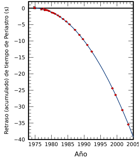
Figura 6.3: Predicción y observación del tiempo en que el pulsar binario de Hulse y Taylor completa cada revolución (tiempo de periastro), respecto al valor newtoniano. Adaptada a partir de esta figura original.
