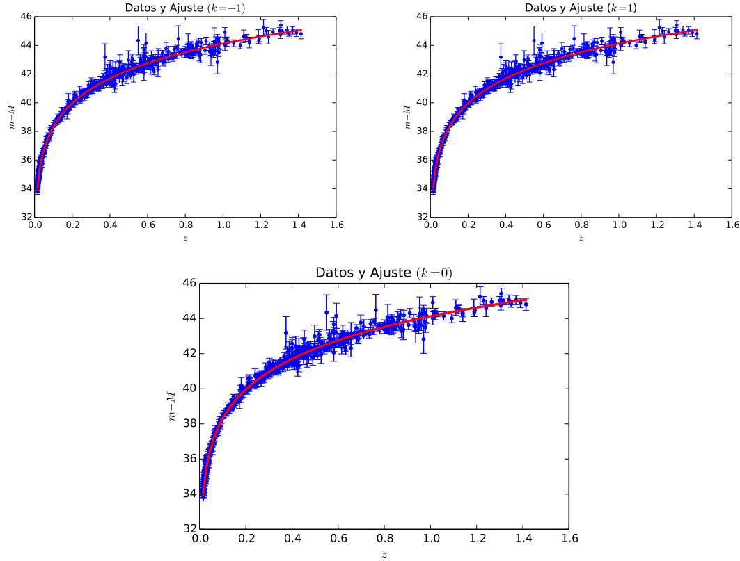
Figura 7.9: El gráfico superior izquierdo corresponde al caso de un universo con curvatura espacial negativa, el superior derecho al caso de un universo con curvatura espacial positiva y el inferior central, al caso de un universo espacialmente plano.
