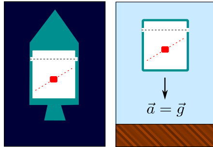
Figura 1.3: Equivalencia entre un SRI en ausencia de gravedad y un SR en caída libre.
