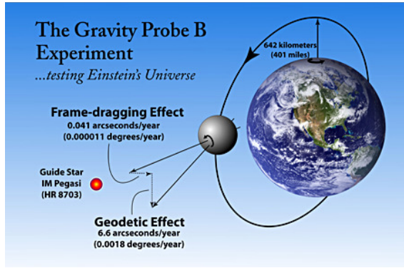
Figura 8.6: Esquema de los ángulos de precesión del giróscopo, medidos por la sonda GPB.
