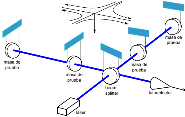
Figura 6.2: Esquema de un detector interferométrico de ondas gravitacionales. Figura original aquí .
