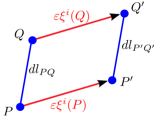
Figura 2.4: Trasladando puntos en la dirección \xi^i(x) .
