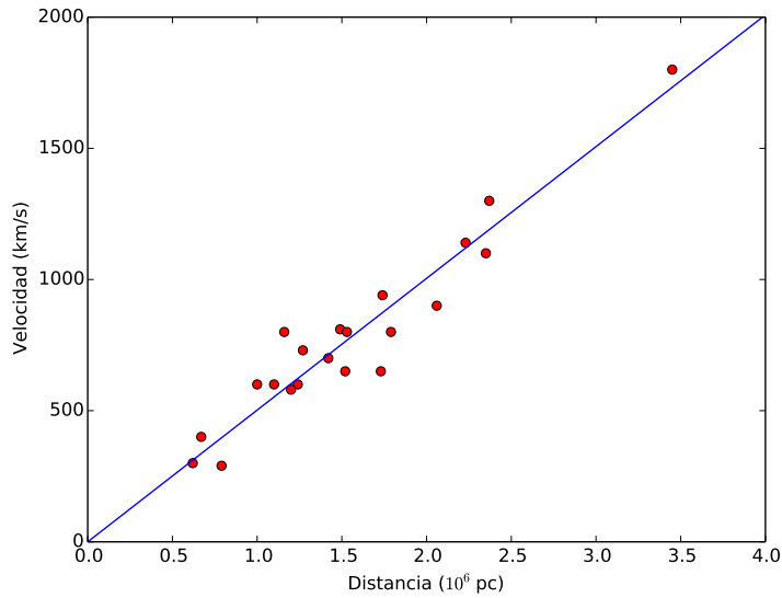
Figura 7.1: Relación entre la velocidad y distancia de las nebulosas, medida por Hubble [?].
