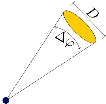
Figura 7.4: El punto azul representa la tierra mientras que el amarillo el objeto en estudio.
