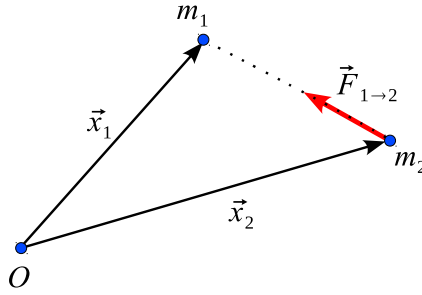
Figura 1.1: Ley de gravitación universal de Newton.
