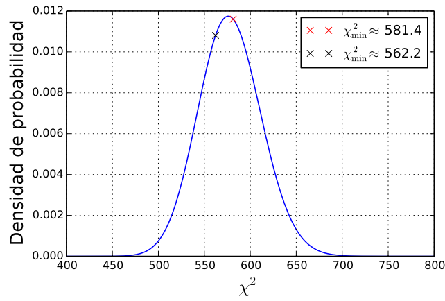
Figura 7.13: Densidad de probabilidad de \chi^2 . Ésta se calculó usando 580 datos y usando dos parámetros libres para ajustar. En el caso de la aproximación en z los parametros son h y q_0 . Por otro lado, para la expresión completa, se fijaron h y \Omega_k en los valores que minimizan \chi^2 , \Omega_M y \Omega_R fueron los considerados como parámetros a ajustar. La x roja corresponde al valor de \chi^2_{\min} con la aproximación a segundo orden en z y la x negra corresponde al valor \chi^2_{\min} usando la expresión completa. El valor óptimo de \chi^2 según su distribución de probabilidad es de aproximadamente 576.9.
