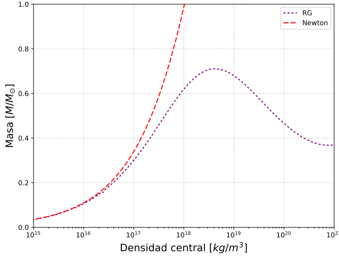
Figura 10.3: Relación masa-densidad central para estrellas de neutrones con las ecuaciones TOV y newtonianas
