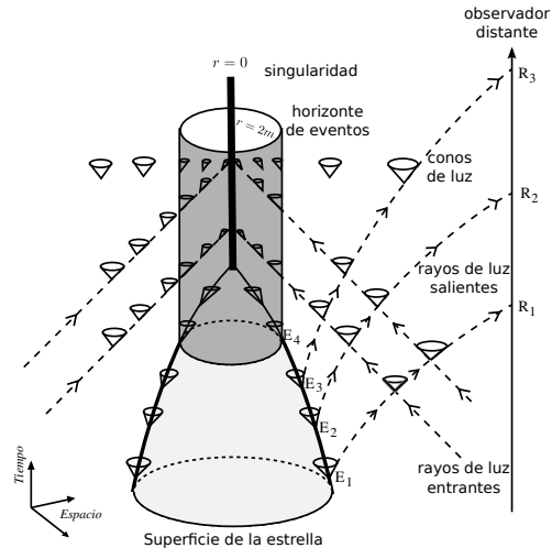
Figura 4.3: Colapso estelar, figura adaptada a partir de Ref. [43]
