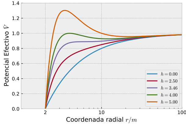
Figura 3.1: Potencial Efectivo (escala logarítmica en r ).
