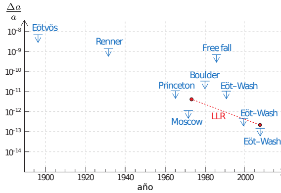
Figura 1.2: Límites a posibles violaciones del PED. Figura adaptada a partir de la original en [4].
