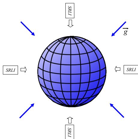
Figura 1.5: Sistemas de referencia localmente inerciales cayendo hacia la Tierra.
