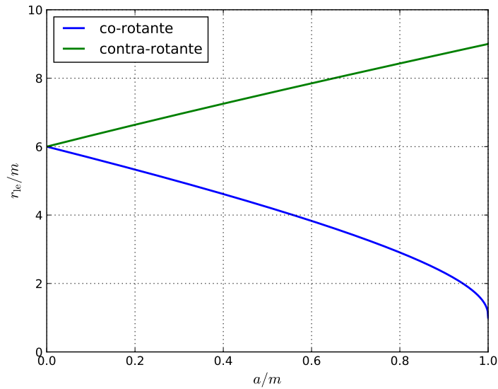
Figura 5.10: Radios de última órbita circular ecuatorial estable.
