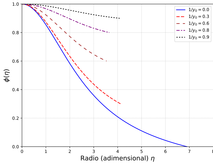
Figura 9.2: Soluciones \phi(\eta) de la ecuación de estructura de Fermi.
