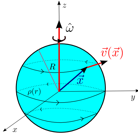
Figura 8.1: Modelo de fuente de campo gravitacional: Una distribución de masa esféricamente simétrica que rota, uniforme- y lentamente, en torno a un eje fijo.
