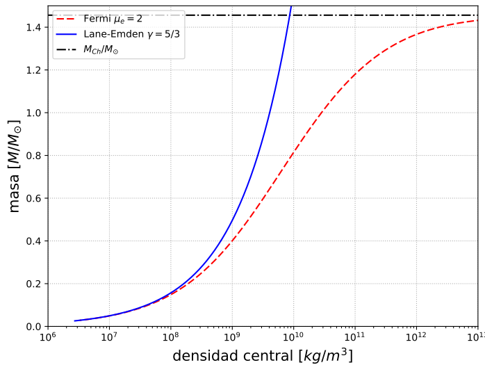
Figura 9.4: Relación masa-densidad central para enanas blancas compuestas un gas de electrones completamente degenerado en los casos límite no relativista ( \gamma = 5/3 ) y ultra relativista ( \gamma = 4/3 ).
