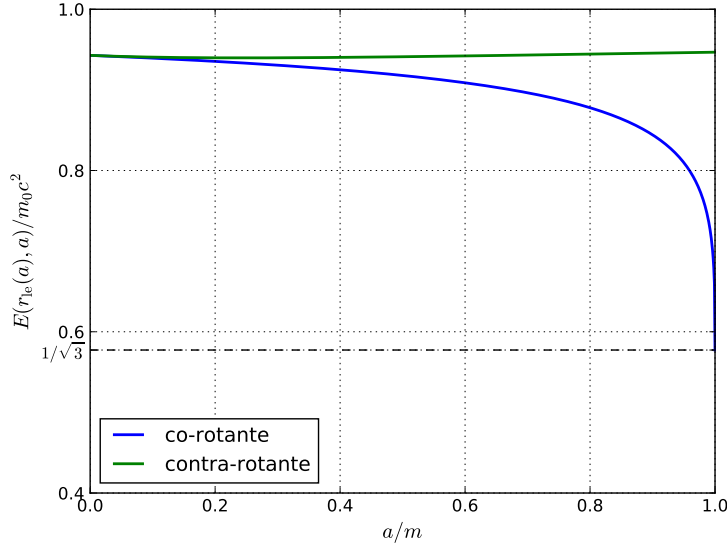
Figura 5.11: Energía de la última órbita circular ecuatorial estable.
