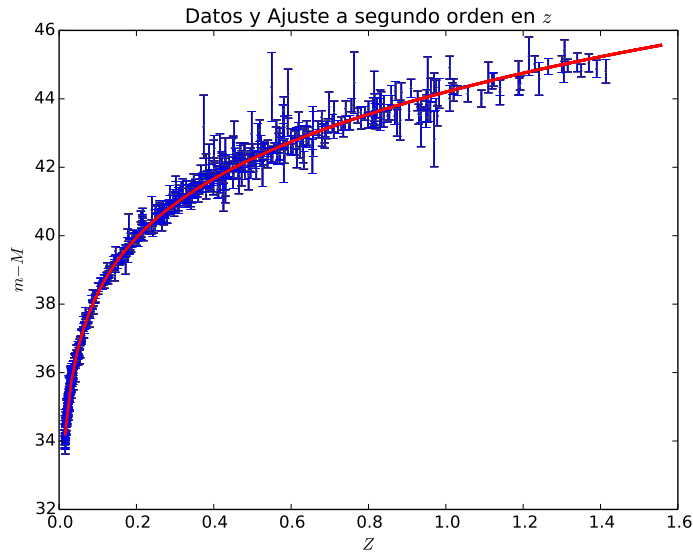
Figura 7.7: Gráfico correspondiente al ajuste de la expresión a segundo orden en z . Con h = 0.688 y q_0 = -0.175 .
