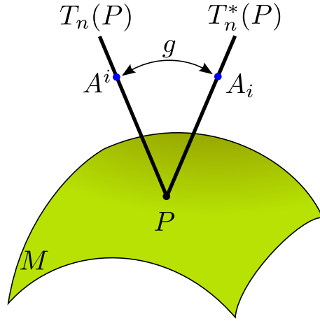
Figura 2.3: El tensor métrico define una relación uno a uno (isomorfismo) entre los espacios tangente y cotangente en cada punto de la variedad.
