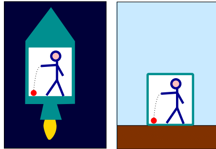
Figura 1.4: Equivalencia entre campo gravitacional y aceleración.
