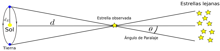
Figura 7.2: El movimiento de la Tierra alrededor del Sol.
