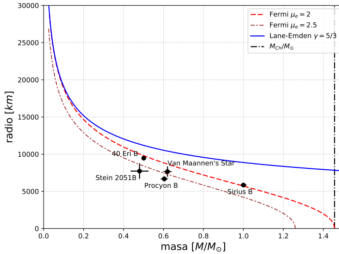
Figura 9.3: Relación masa-radio para enanas blancas compuestas un gas de electrones completamente degenerado en los casos límite no relativista ( \gamma = 5/3 ) y ultra relativista ( \gamma = 4/3 ).
