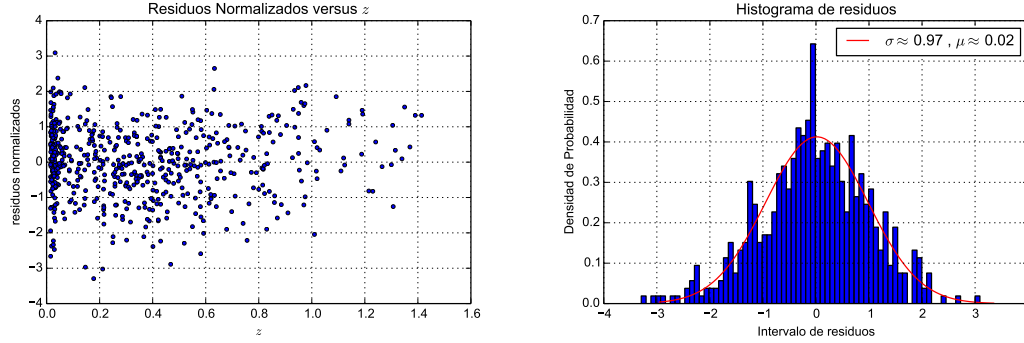
Figura 7.8: El gráfico de la izquierda corresponde al diagrama de residuos del ajuste, mientras que el de la derecha corresponde al histograma de residuos al cual se le ajustó una curva gaussiana, con \sigma^2 la varianza y \mu la media.
