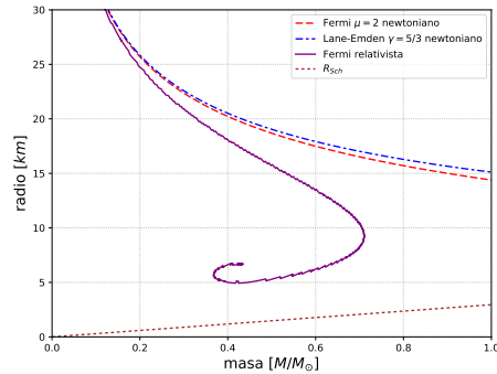
Figura 10.5: Relación Masa-Radius para estrellas de neutrones con las ecuaciones TOV y newtonianas
