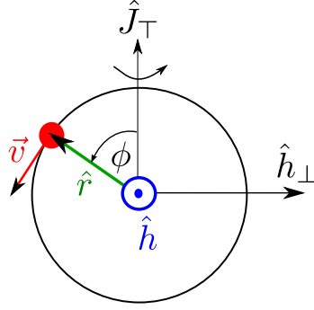
Figura 8.5: Giróscopo en una órbita circular polar en torno a la Tierra.
