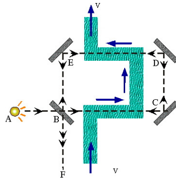
Figura 5.8: Diagrama del interferómetro de Fizeau
