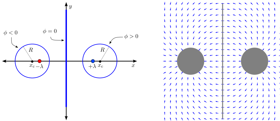
Figura 1.15: Superficies equipotenciales y líneas de campo. Código Python de la figura de la derecha disponible aquí .
