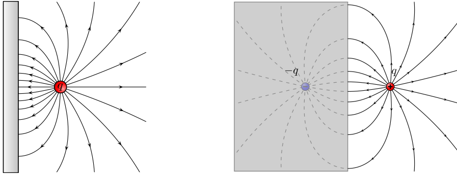
Figura 1.11: Campo eléctrico de plano conductor (puesto a Tierra) y carga puntual. Figuras adaptadas de este y este archivo original.
