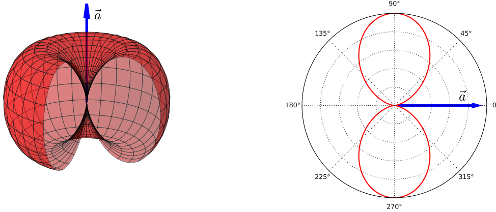
Figura 4.4: Distribución de potencia para una carga no-relativista en movimiento acelerado. Códigos Python aquí y aquí .
