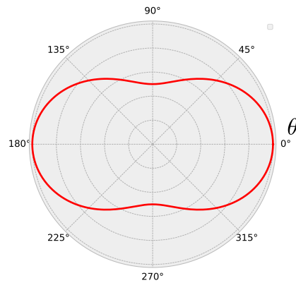
Figura 4.9: Sección diferencial de scattering de Thomson. Código Python aquí .
