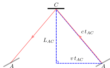
Figura 5.2: Propagación en el segunda brazo, respecto a un SR comóvil con el éter.
