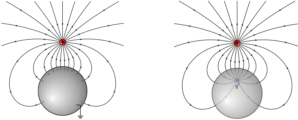
Figura 1.13: Campo eléctrico de esfera conductora (puesta a Tierra) y carga puntual. Figuras adaptadas a partir de este y este archivo original.
