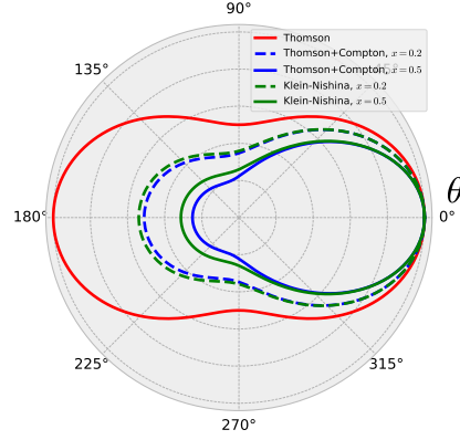
Figura 4.10: Sección diferencial de scattering Thomson (4.169) y correcciones cuántico-relativistas (4.170). El gráfico muestra d\sigma/d\Omega en función de \theta para distintos valores de x := \hbar\omega/mc^2 .
