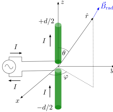
Figura 4.14: Esquema para antena lineal.
