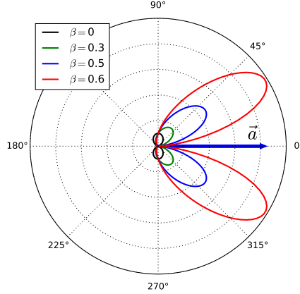
Figura 4.7: Lóbulos de radiación para una carga relativista acelerada. Suponemos iguales aceleraciones y normalizamos con respecto a \mu q^2 \vec{a}^2 / 16\pi^2 c . Código Python aquí .
