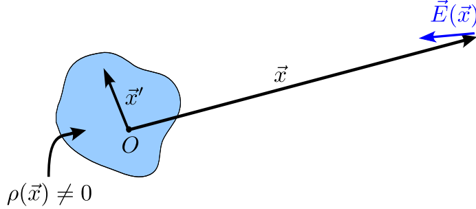
Figura 1.17: Esquema de la expansión multipolar eléctrica.
