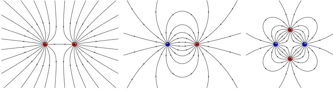
Figura 1.2: Ejemplos simples de líneas de campo eléctrico.
