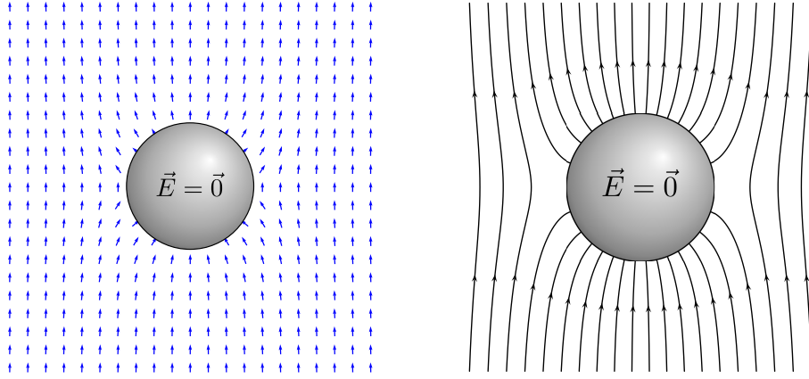
Figura 1.9: Campo eléctrico de una esfera conductora neutra en un campo eléctrico externo. El gráfico de la izquierda (normalizado) fue creado usando este script Python. La figura de la derecha fue generada usando VectorFieldPlot , a partir de este archivo original.
