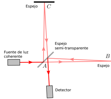
Figura 5.1: Esquema del interferómetro
