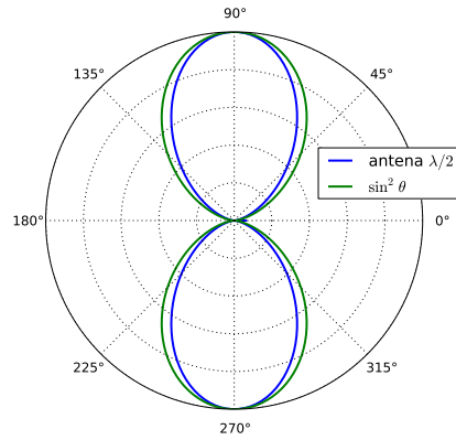
Figura 4.15: Lóbulo de radiación para la antena de media onda en el plano xz .
