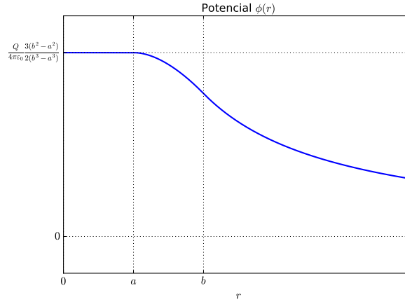
Figura 1.5: Potencial eléctrico como función del radio.
