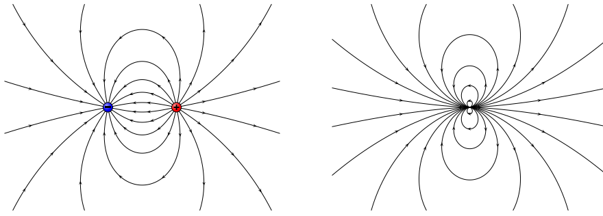
Figura 1.18: Dipolo (dos cargas opuestas) versus dipolo ideal. Figuras creadas usando VectorFieldPlot [1].
