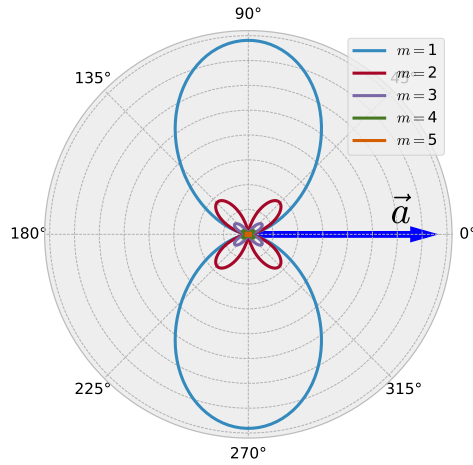
Figura 4.11: Lóbulo de radiación para m = 1, \dots, 5 , \beta = 0.5 . Código Python aquí .
