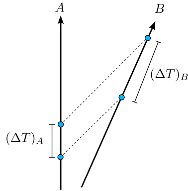
Figura 5.5: Dos observadores inerciales intercambiando señales luminosas.
