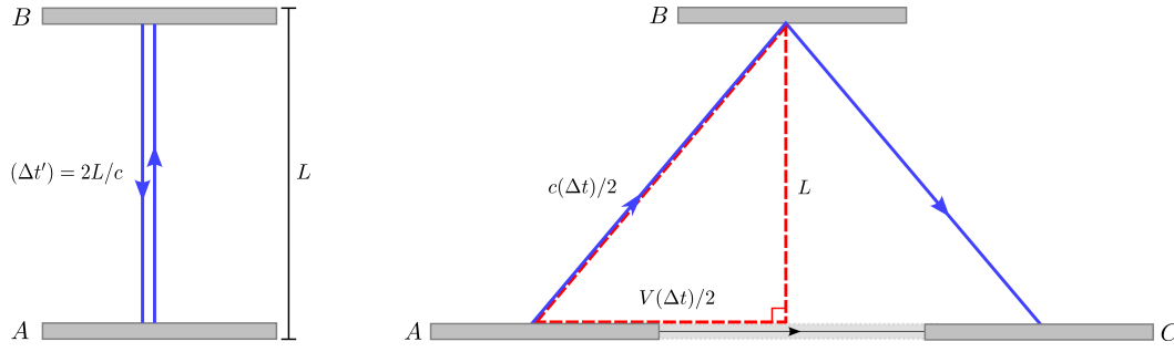
Figura 5.13: Dilatación del tiempo en el “reloj de luz”. Izquierda: SRI comóvil K' . Derecha: SRI K respecto al cual el reloj se mueve con velocidad v = \beta c . Figuras adaptadas a partir de esta y esta figura original.
