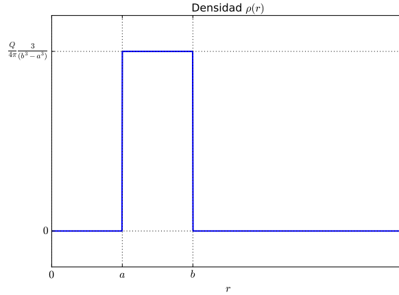
Figura 1.3: Densidad volumétrica como función del radio.
