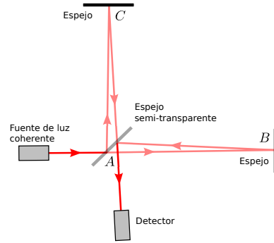
Figura 5.1: Esquema del interferómetro
