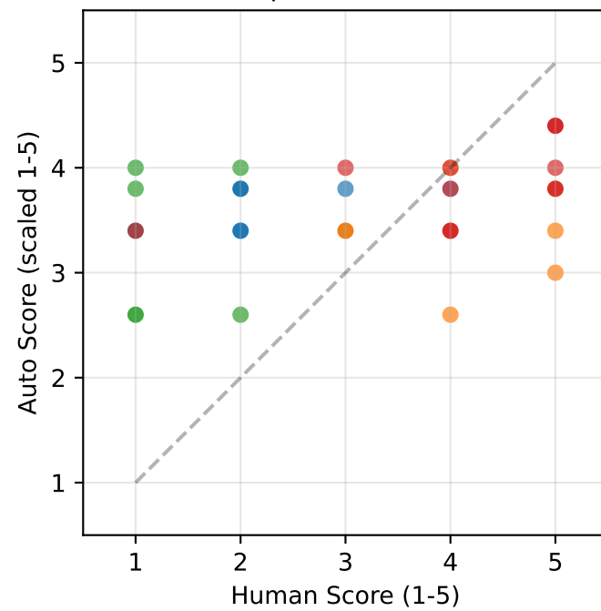
M2.5: Role Adherence \rho=0.107 n.s.
