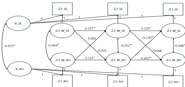
<그림 2> 고등학교 3시점 자아존중감과 학업무기력 RI-CLPM 모형
