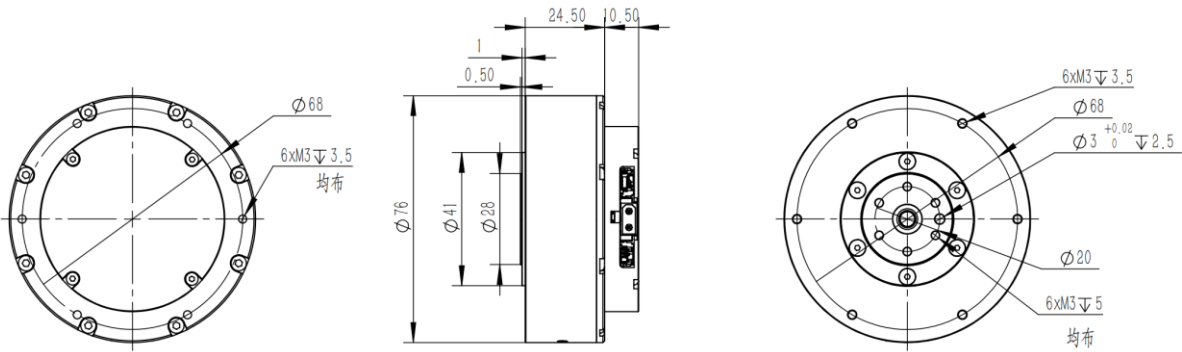
尺寸图
