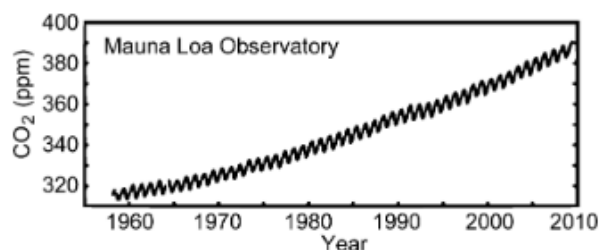
FIGURE 1.5 – Courbe de Keeling Cette courbe représente la mesure de la concentration atmosphérique de CO 2 dans l'atmosphère, au niveau du laboratoire de Mauna Loa. Elle a permis d'identifier l'augmentation de la concentration de ce gaz à effet de serre dans l'atmosphère. Source : HARRIS (2010)
