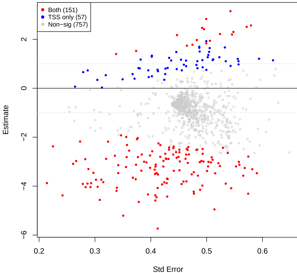
mage vs you – CLR(const=-0.9) (TSS sig overlay)
