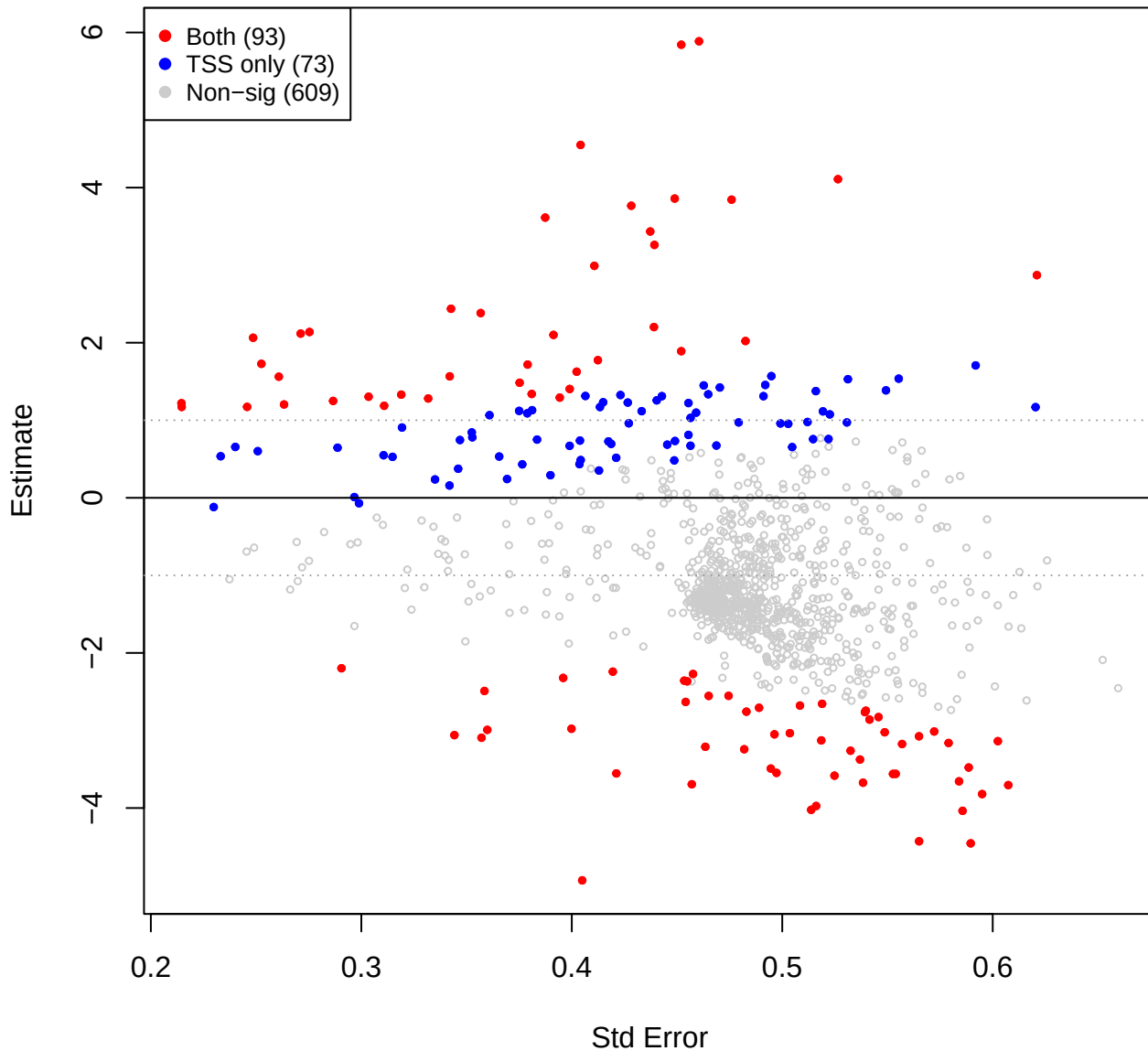
eld vs mid – CLR(const=-0.9) (TSS sig overlay)
