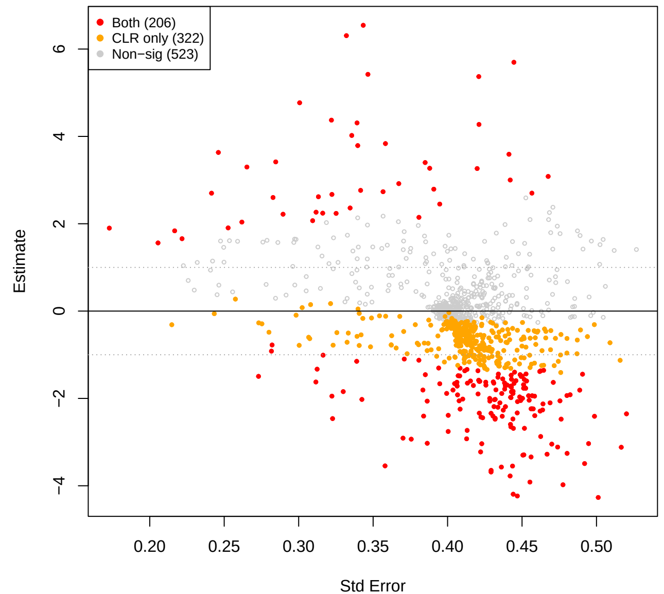
cent vs kin – TSS (CLR(const=-0.9) sig overlay)
