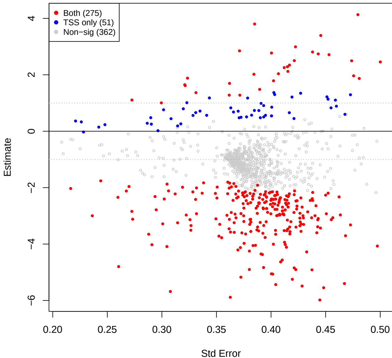
cent vs you - CLR(const=-0.9) (TSS sig overlay)
