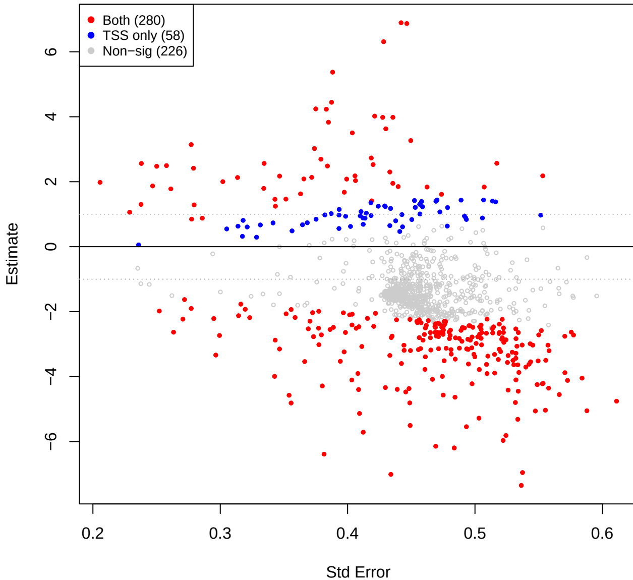
eld vs pup – CLR(const=-0.9) (TSS sig overlay)
