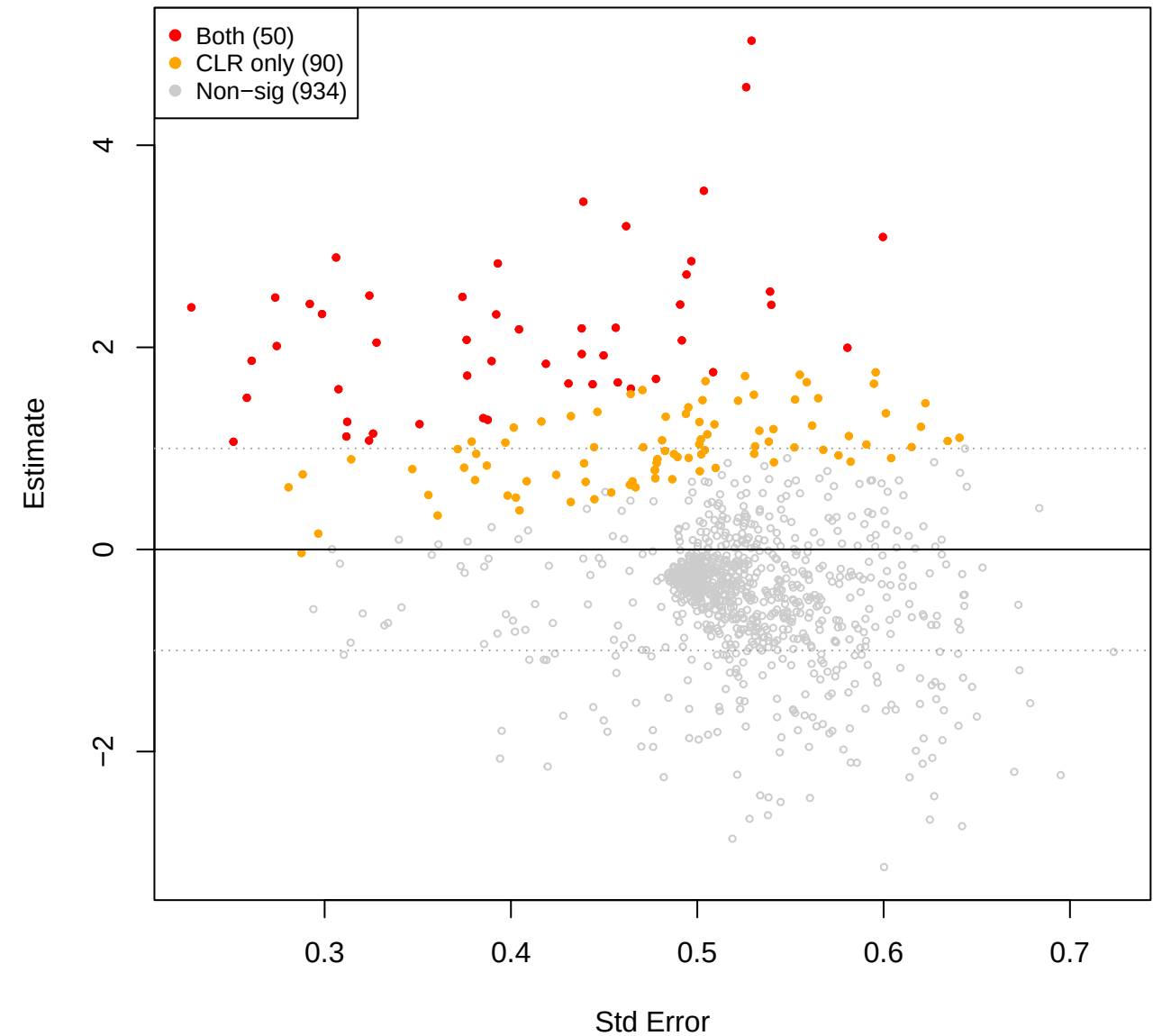
eld vs mage - TSS (CLR(const=0.8) sig overlay)
