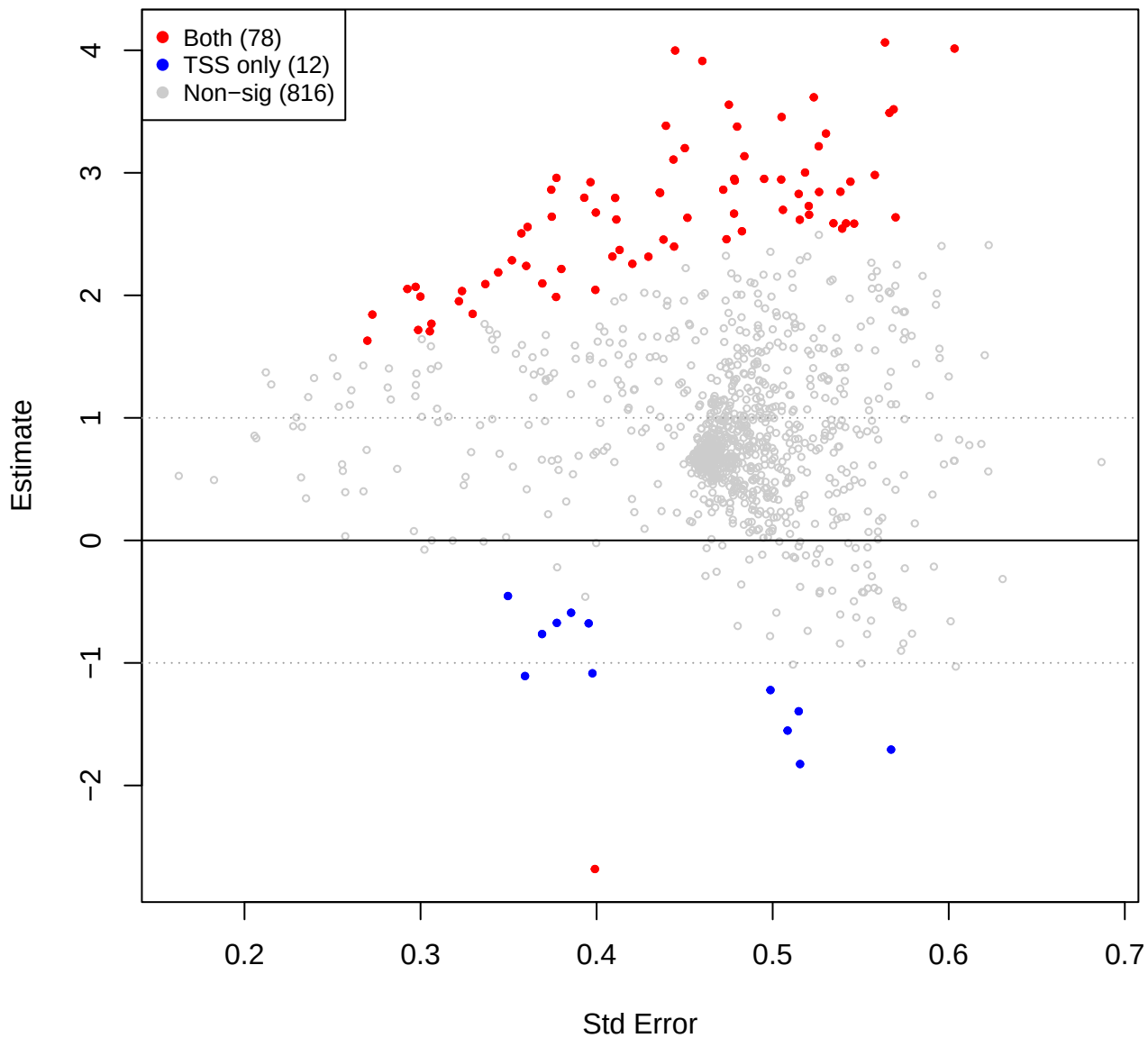
mage vs mid – CLR(const=0.8) (TSS sig overlay)
