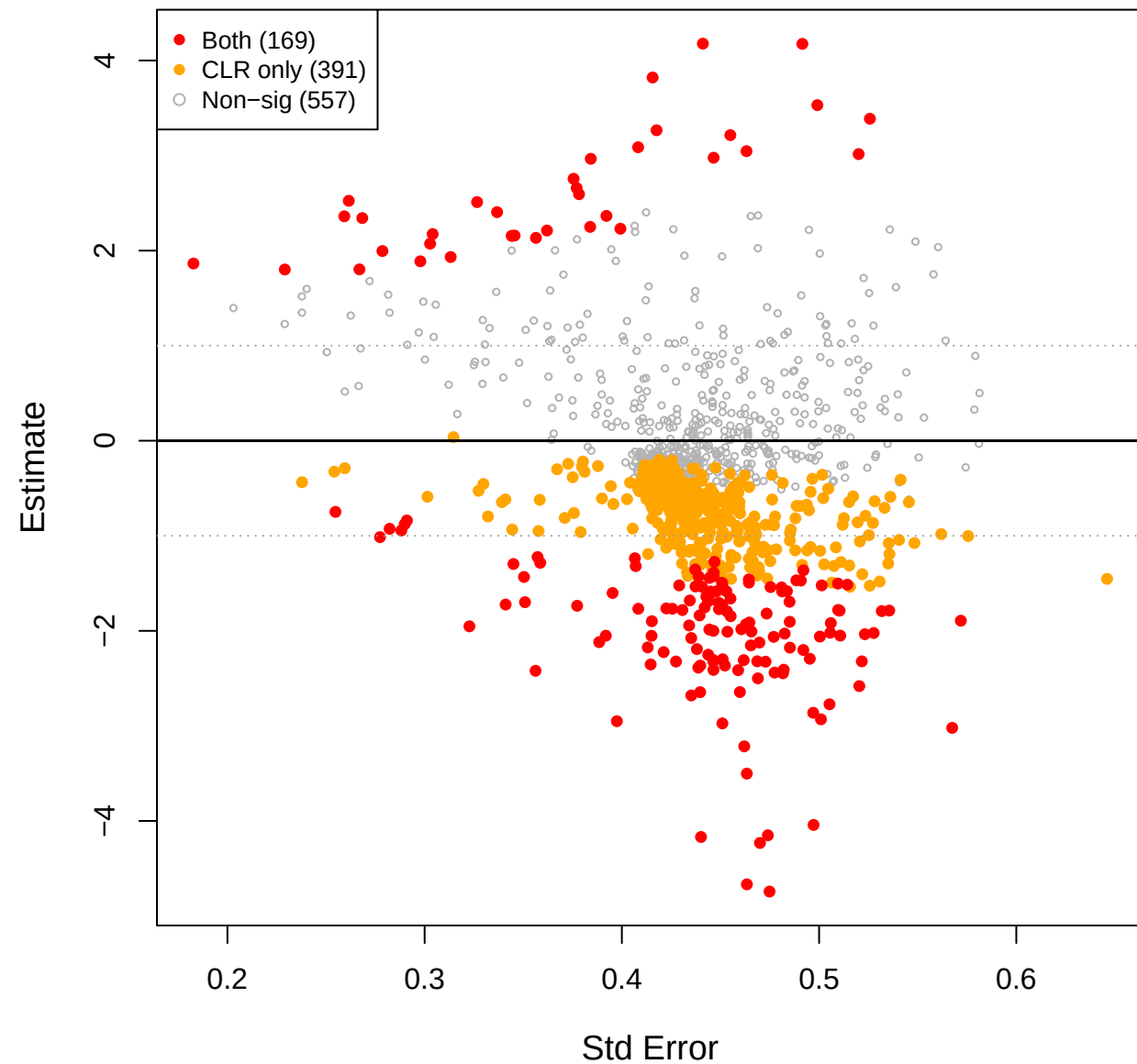
cent vs mage – TSS (CLR(const=-0.8) sig overlay)
