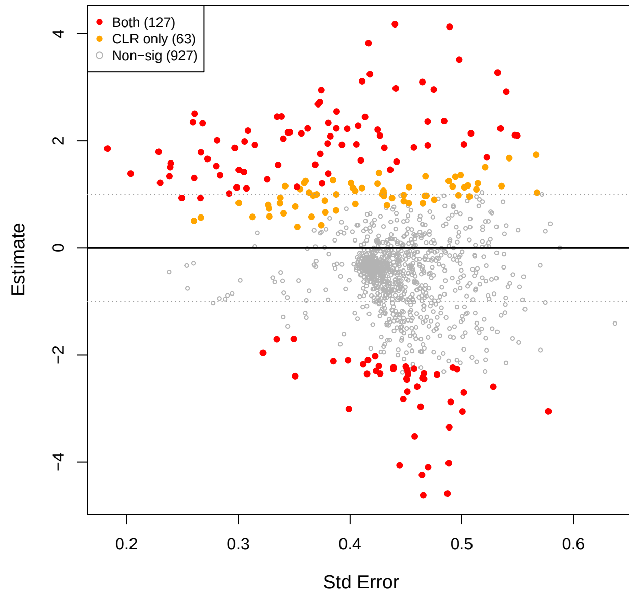
cent vs mage – TSS (CLR(const=0.6) sig overlay)
