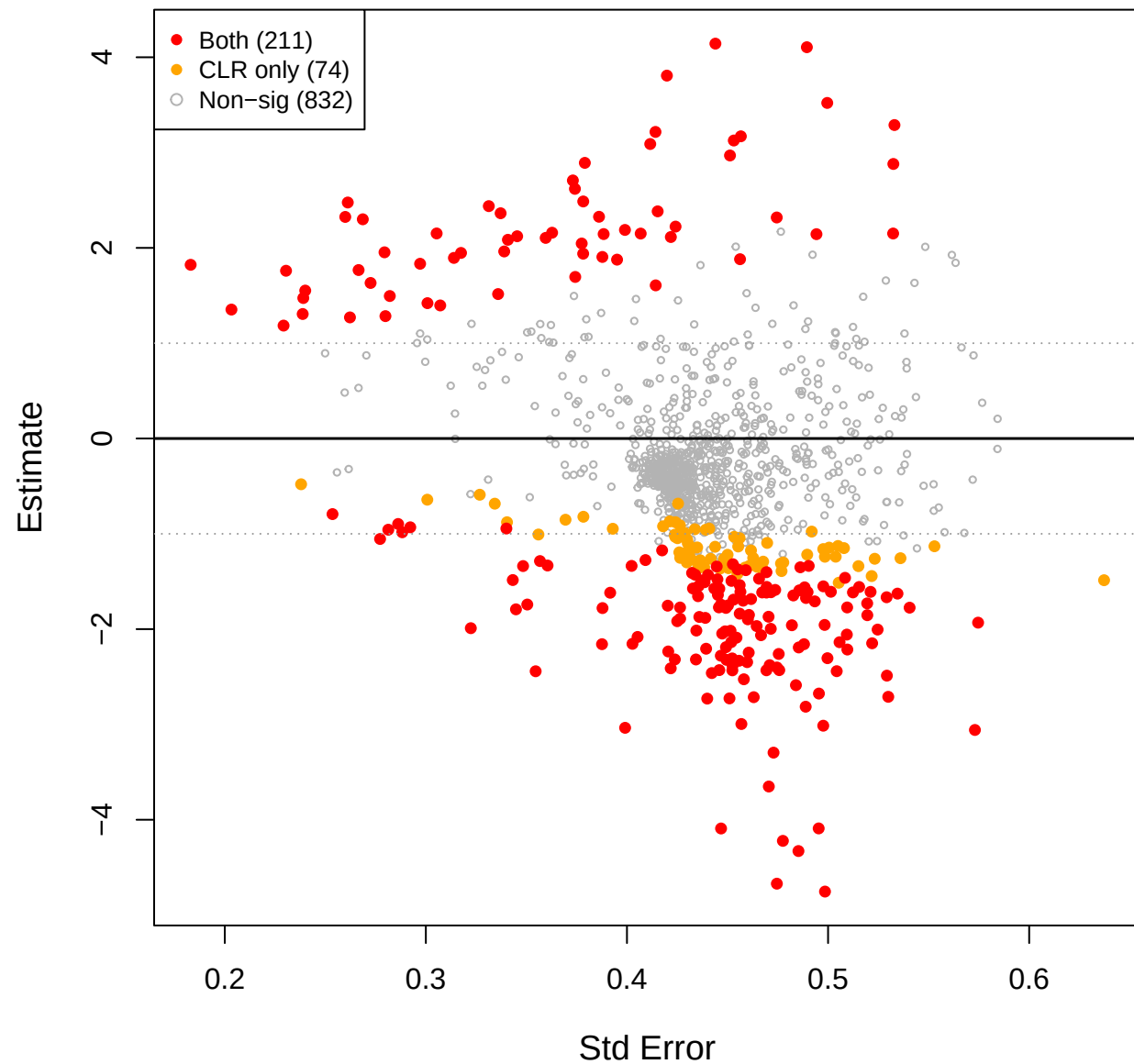
cent vs mage – TSS (CLR(const=-0.3) sig overlay)
