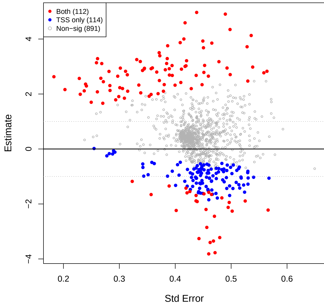
cent vs mage – CLR(const=0.8) (TSS sig overlay)
