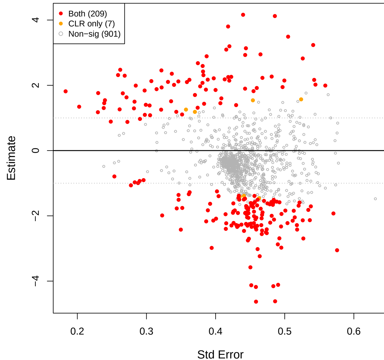
cent vs mage – TSS (CLR(const=0) sig overlay)
