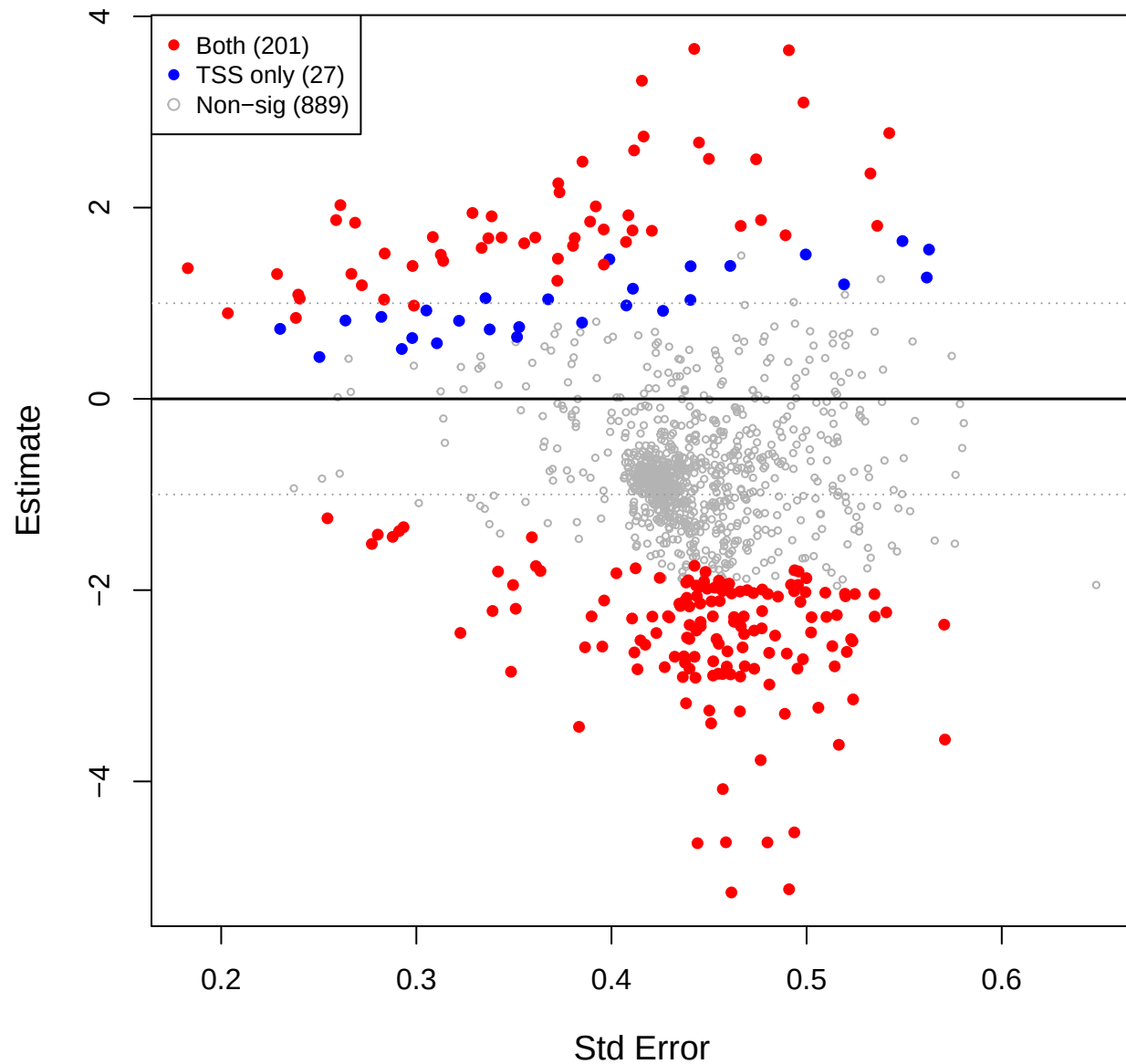
cent vs mage – CLR(const=-0.5) (TSS sig overlay)
