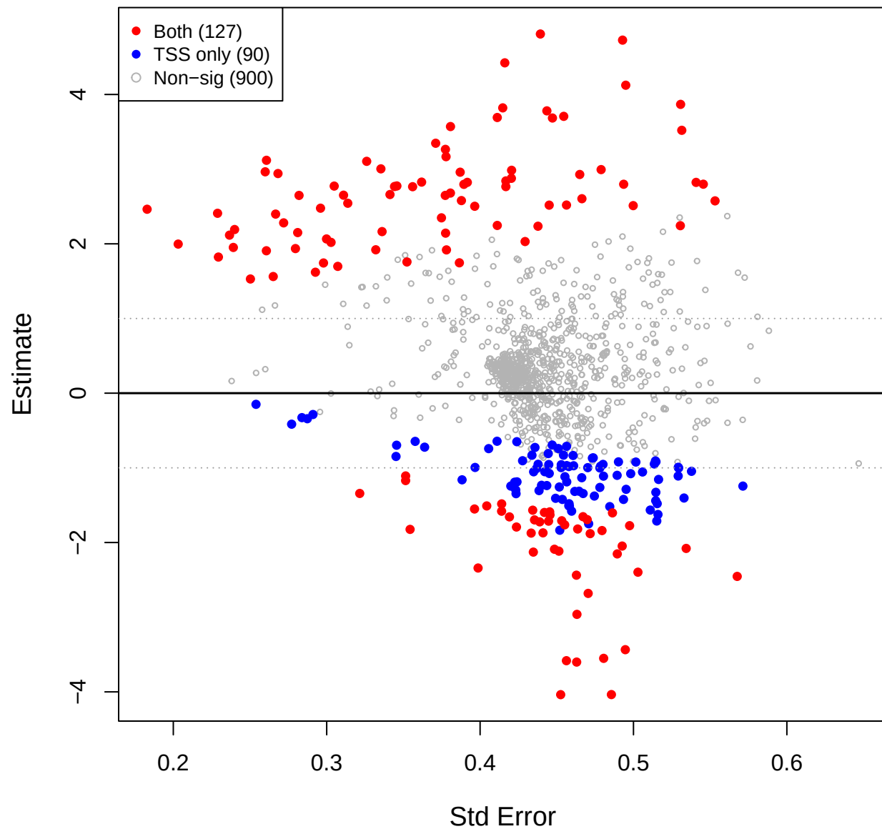
cent vs mage – CLR(const=0.6) (TSS sig overlay)
