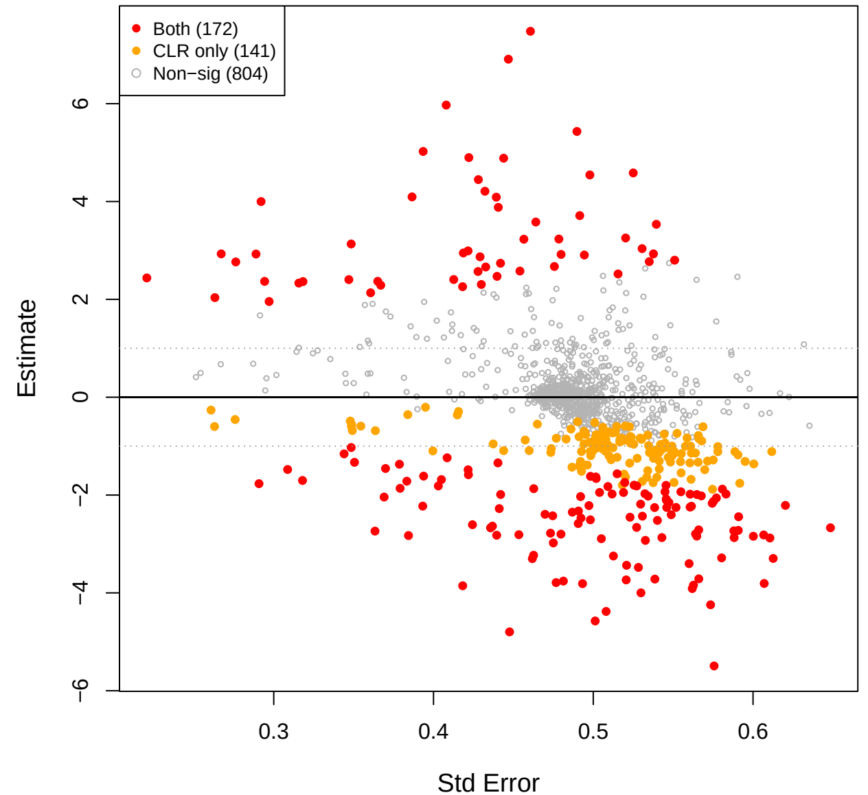
eld vs kin - TSS (CLR(const=-0.8) sig overlay)
