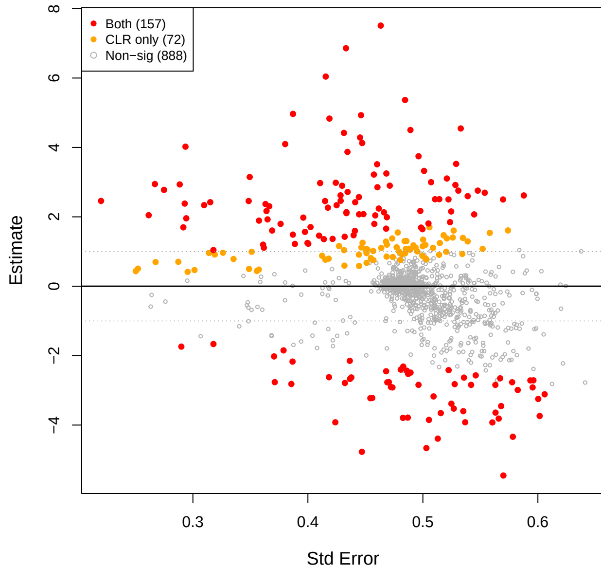
eld vs kin – TSS (CLR(const=0.6) sig overlay)
