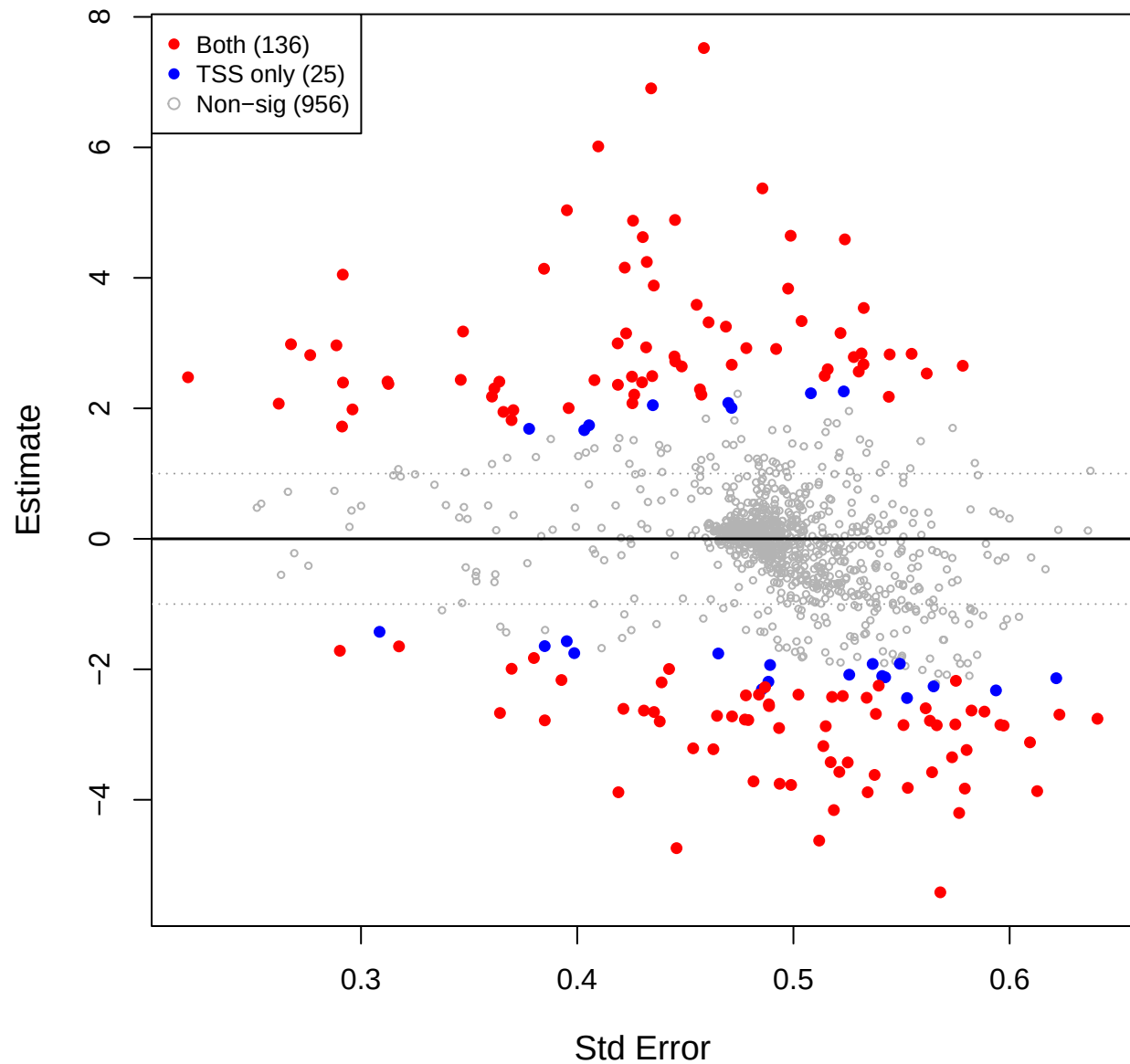
eld vs kin – CLR(const=0) (TSS sig overlay)
