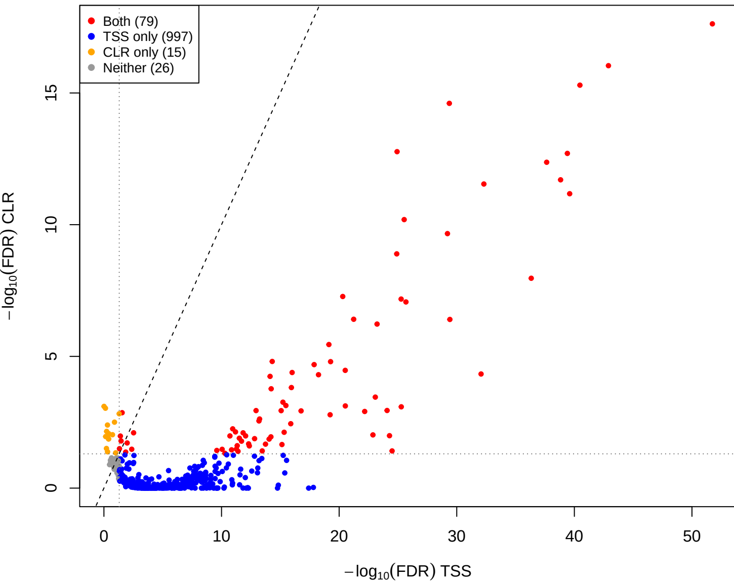
eld vs mage – CLR vs TSS(const=3) (gamma = 1e-05)
