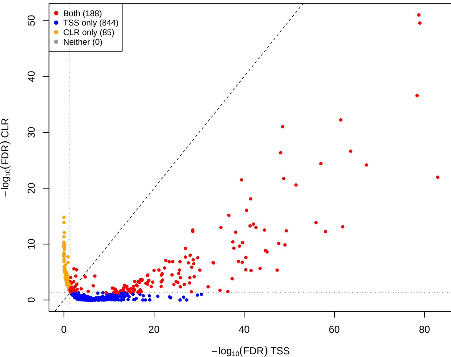
cent vs kin - CLR vs TSS(const=3) (gamma = 1e-05)
