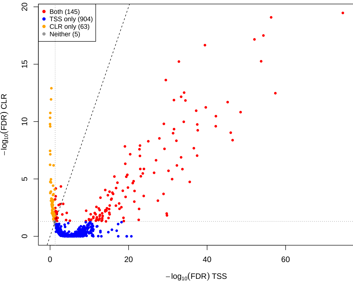
cent vs mage – CLR vs TSS(const=3) (gamma = 1e-05)
