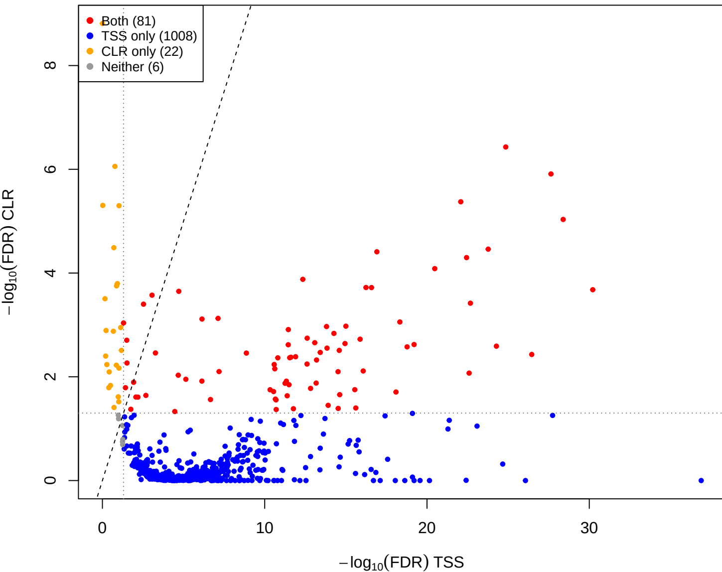
kin vs mage – CLR vs TSS(const=3) (gamma = 1e-05)
