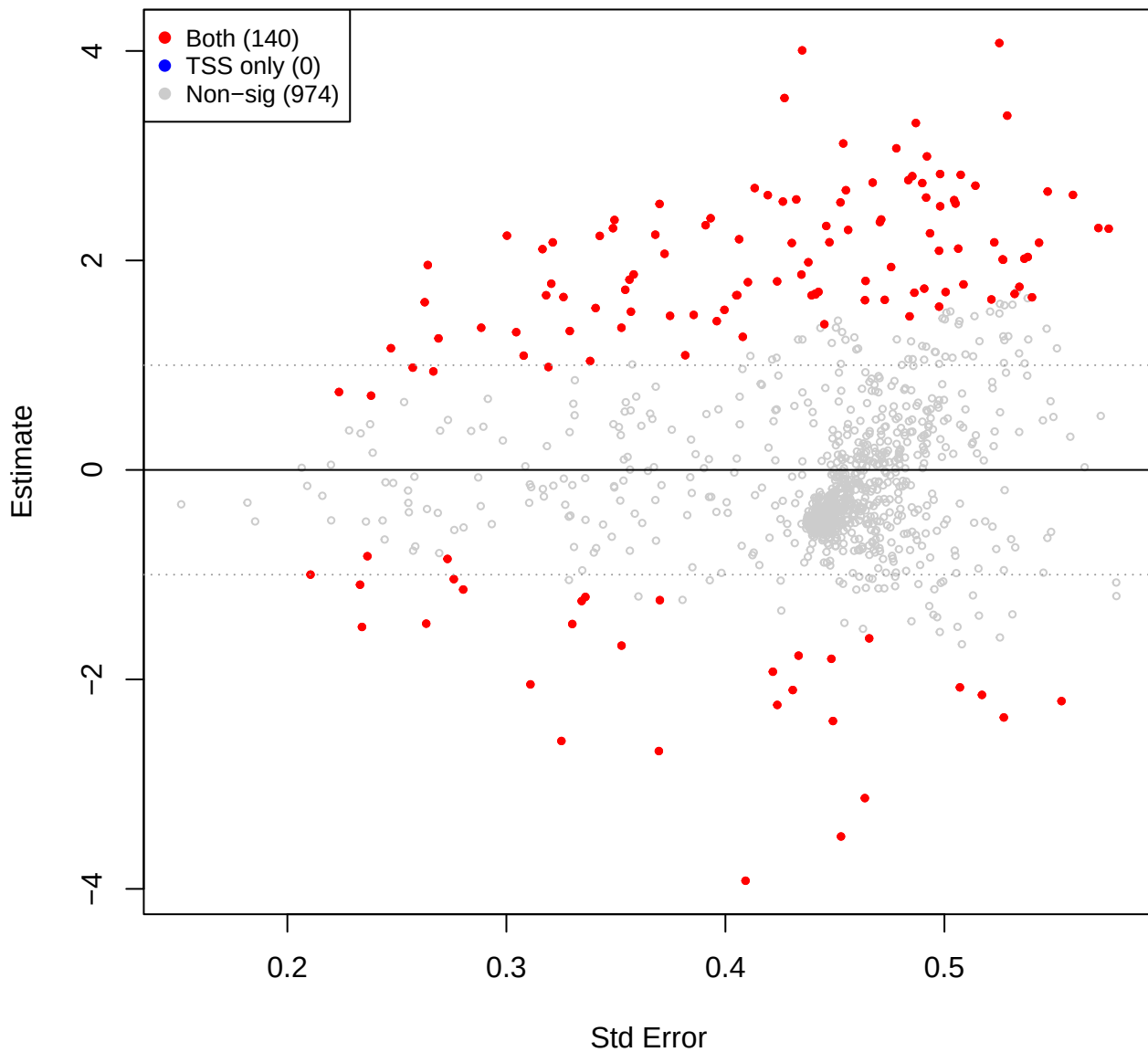
kin vs mid – CLR(const=0) (TSS sig overlay)
