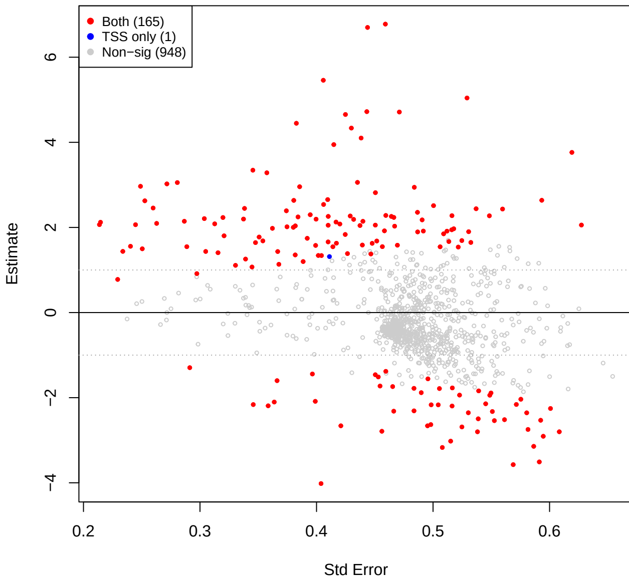
eld vs mid – CLR(const=0) (TSS sig overlay)
