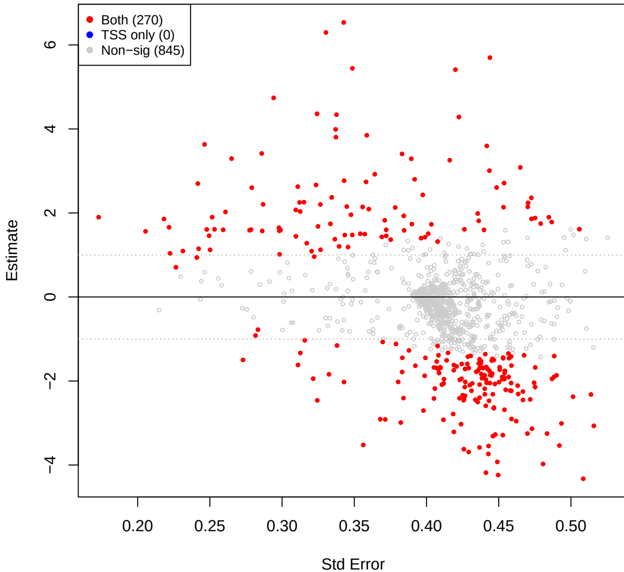
cent vs kin – CLR(const=0) (TSS sig overlay)
