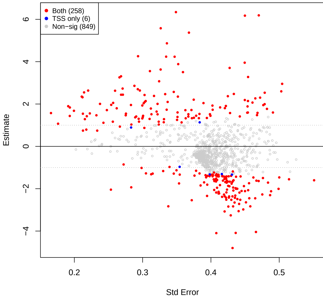
cent vs mid – CLR(const=0) (TSS sig overlay)
