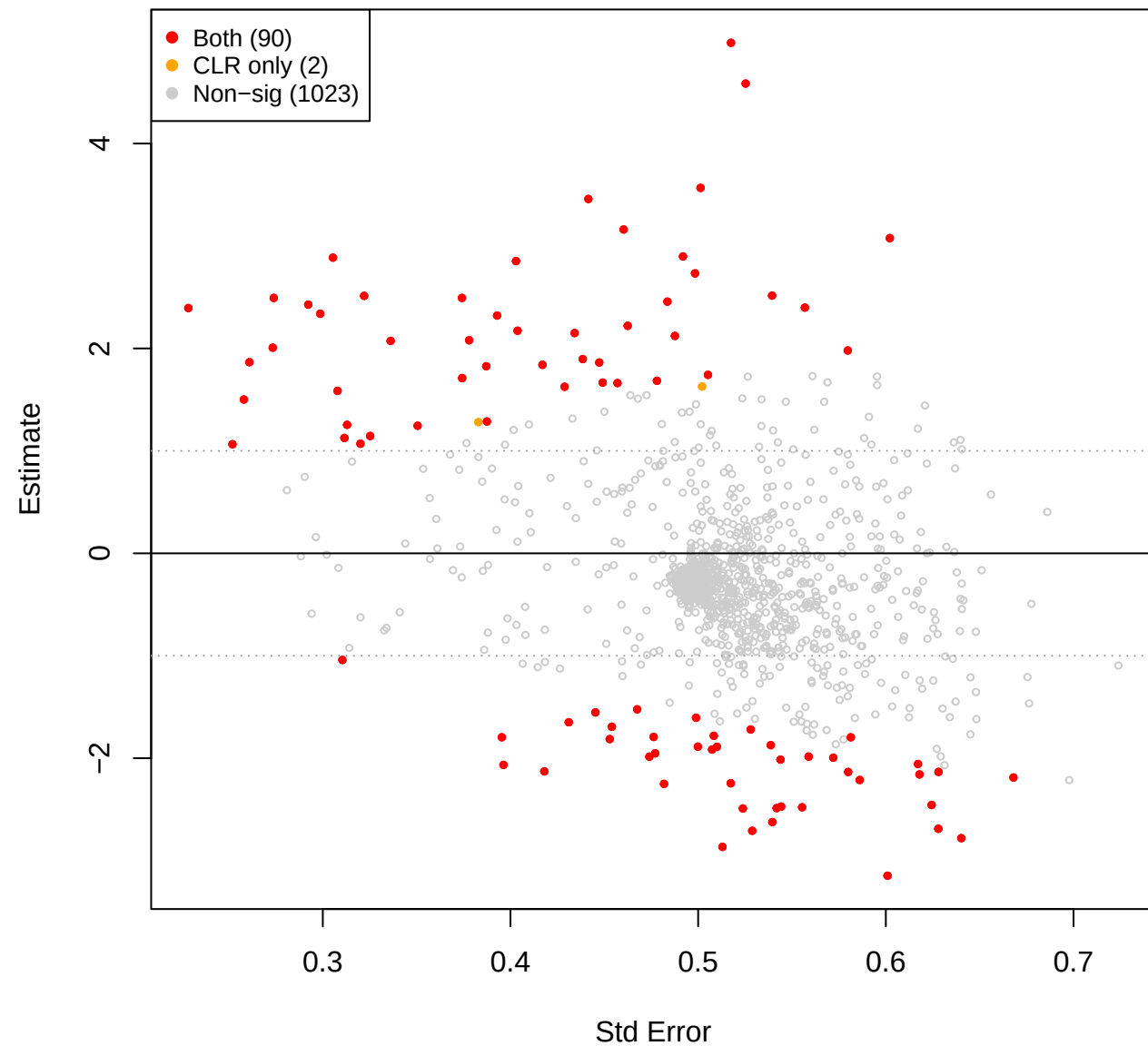
eld vs mage - TSS (CLR(const=0) sig overlay)
