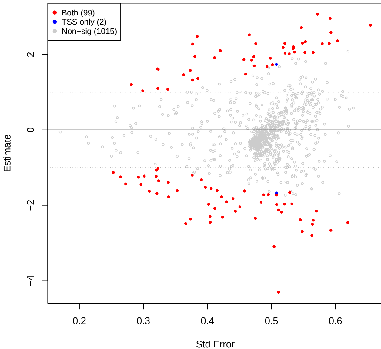
kin vs mage - CLR(const=0) (TSS sig overlay)
