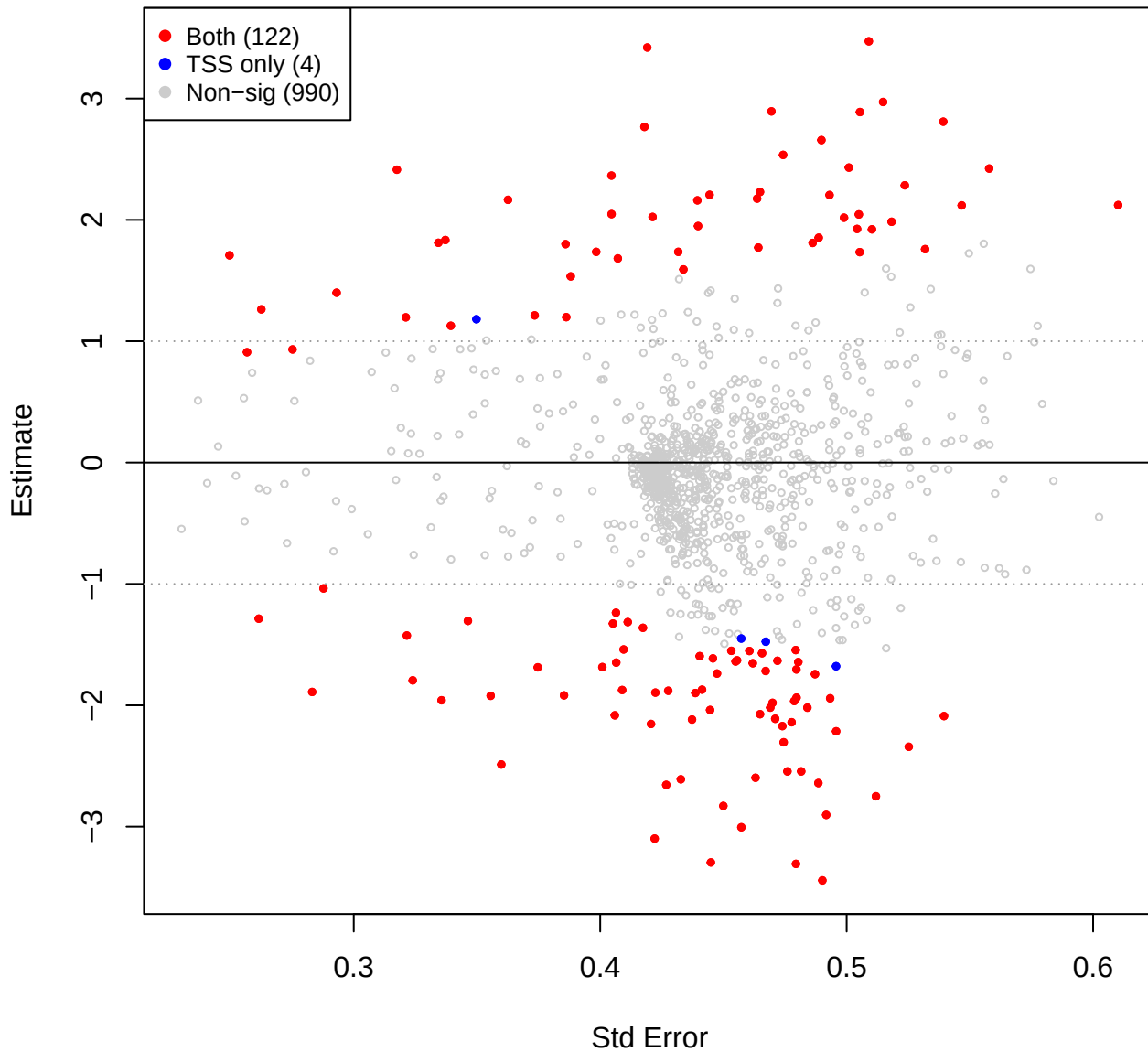
cent vs eld – CLR(const=0) (TSS sig overlay)
