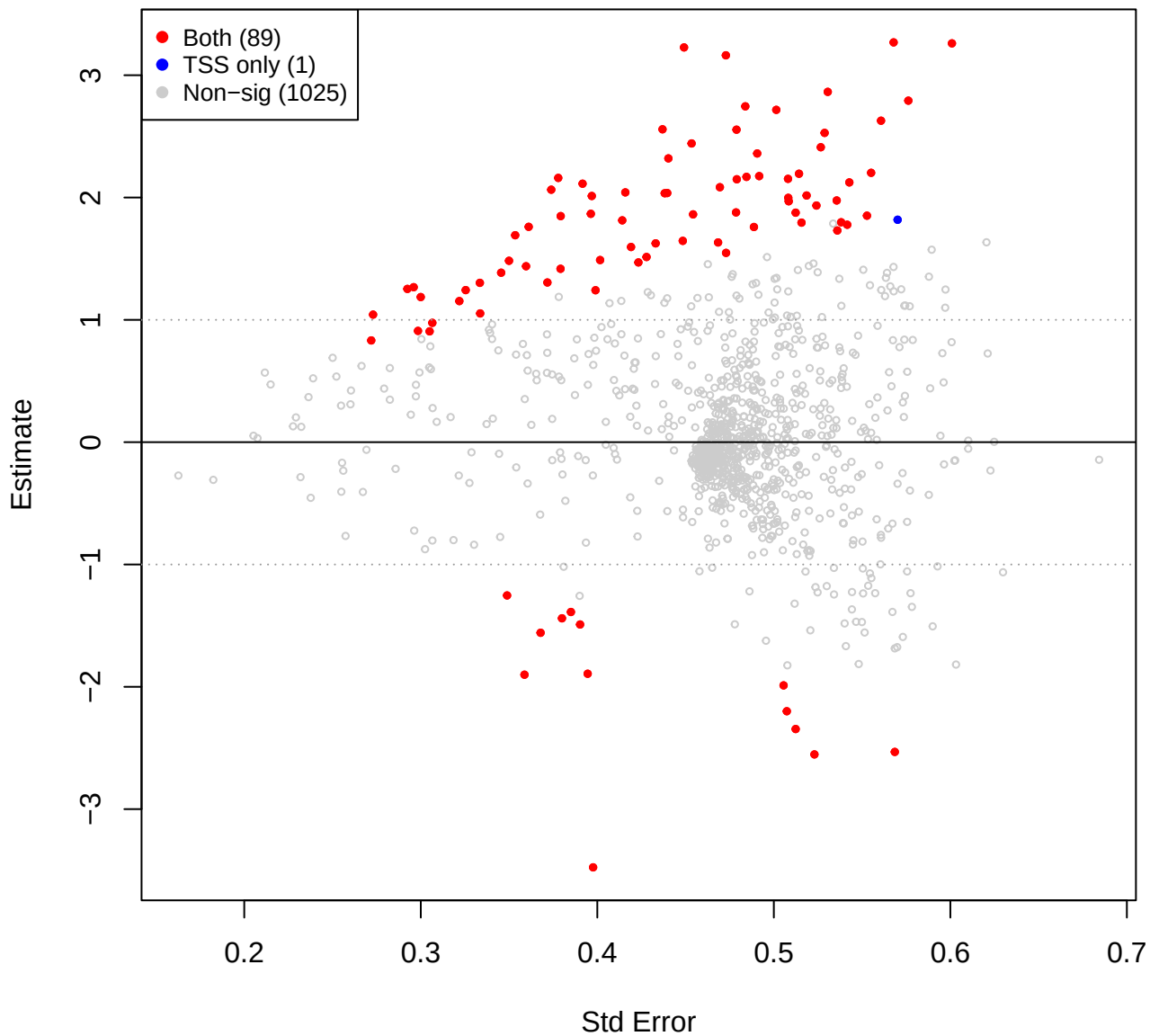
mage vs mid – CLR(const=0) (TSS sig overlay)
