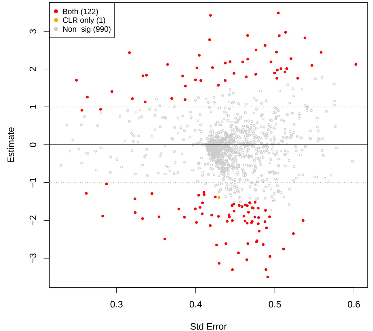
cent vs eld – TSS (CLR(const=0) sig overlay)
