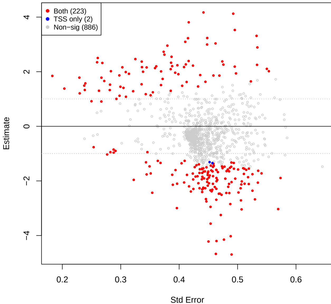
cent vs mage – CLR(const=0) (TSS sig overlay)
