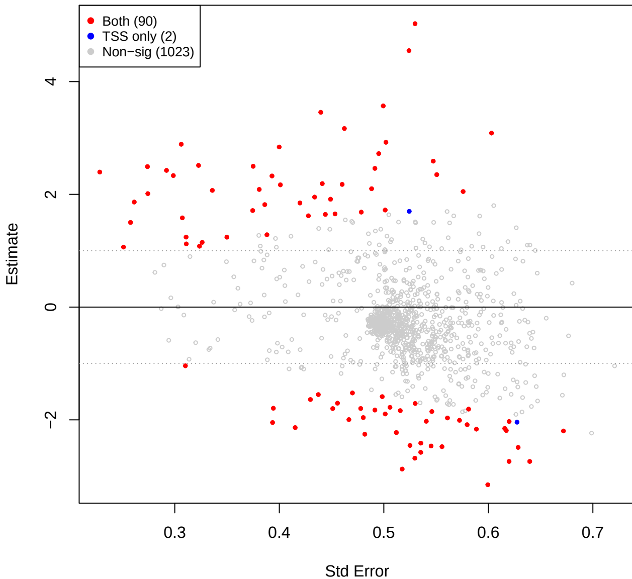
eld vs mage - CLR(const=0) (TSS sig overlay)
