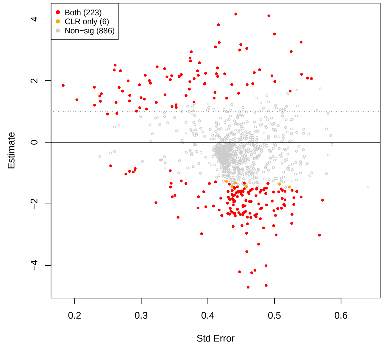
cent vs mage – TSS (CLR(const=0) sig overlay)
