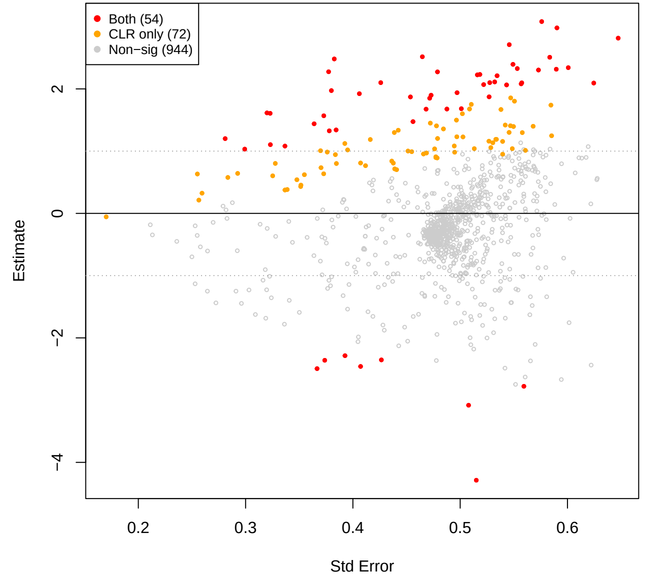
kin vs mage - TSS (CLR(const=0.6) sig overlay)
