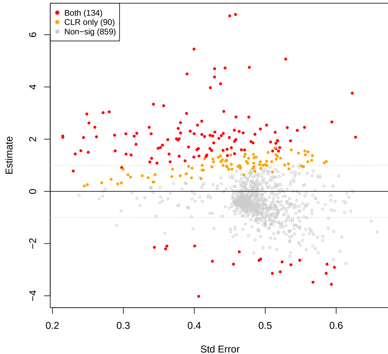
eld vs mid – TSS (CLR(const=0.6) sig overlay)
