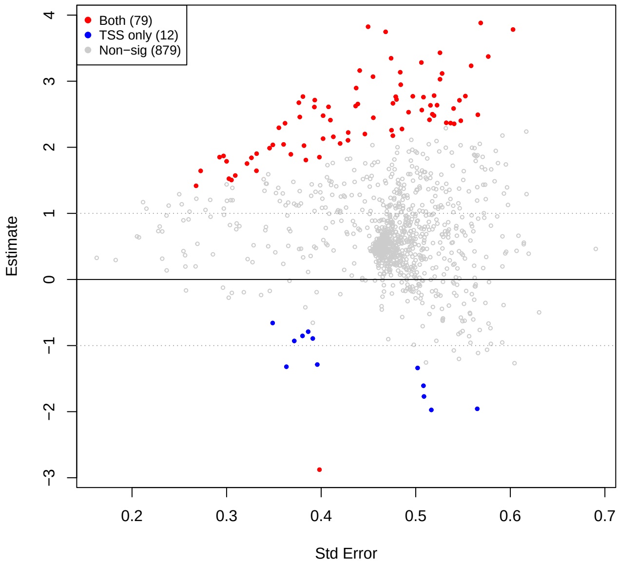
mage vs mid – CLR(const=0.6) (TSS sig overlay)
