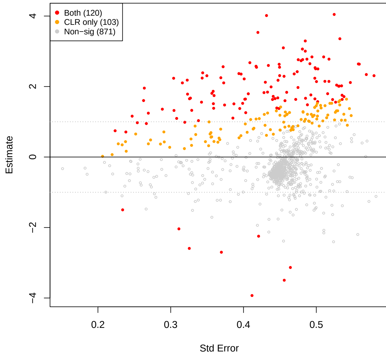
kin vs mid - TSS (CLR(const=0.6) sig overlay)
