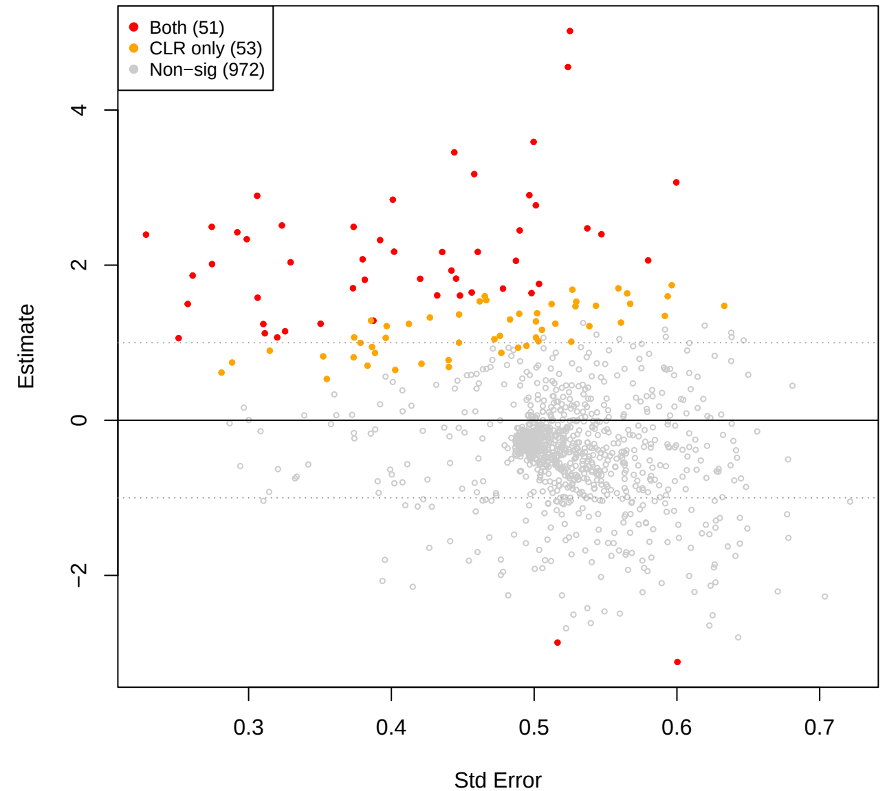
eld vs mage - TSS (CLR(const=0.6) sig overlay)
