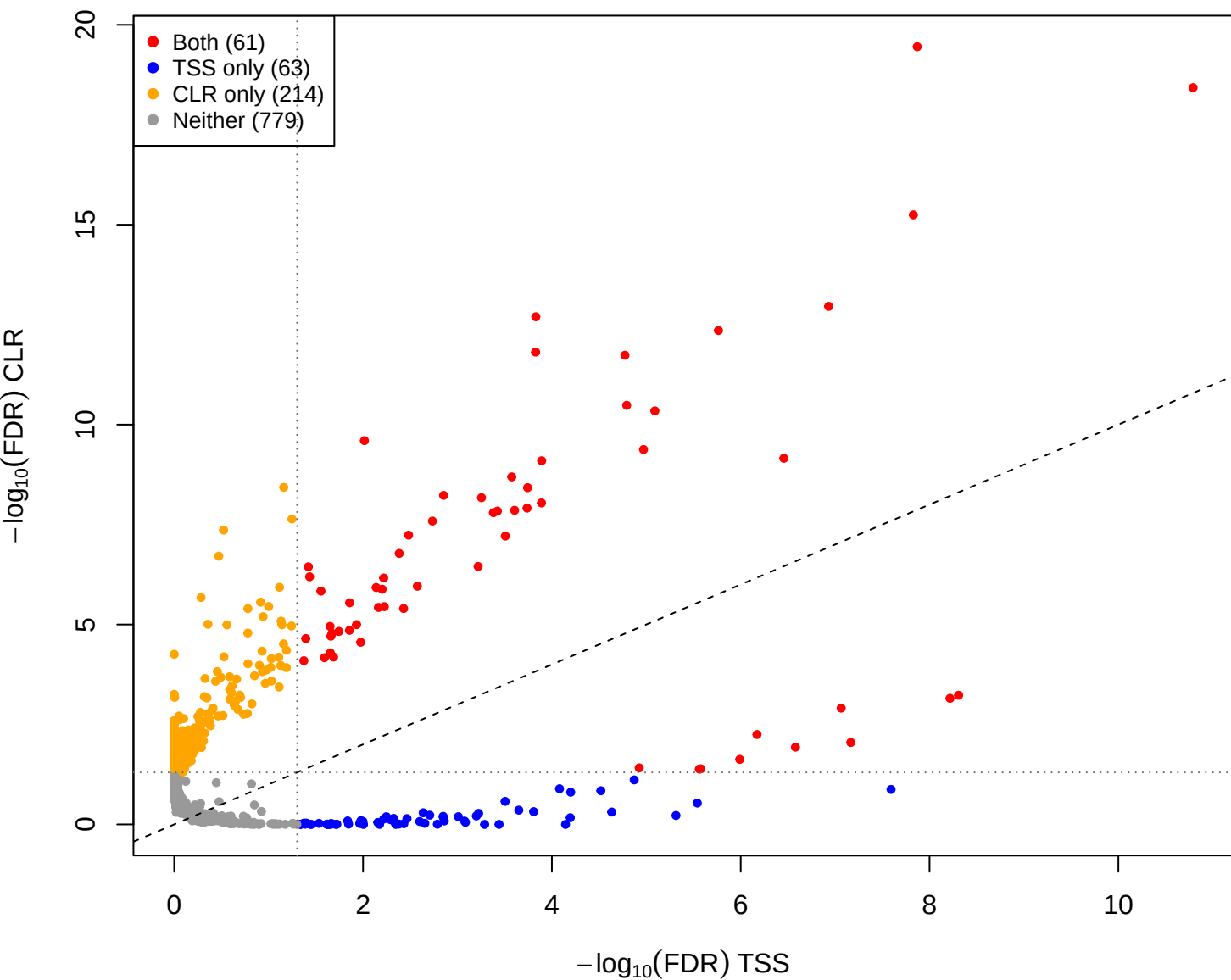
cent vs eld - CLR(const=1) vs TSS (gamma = 1e-05)
