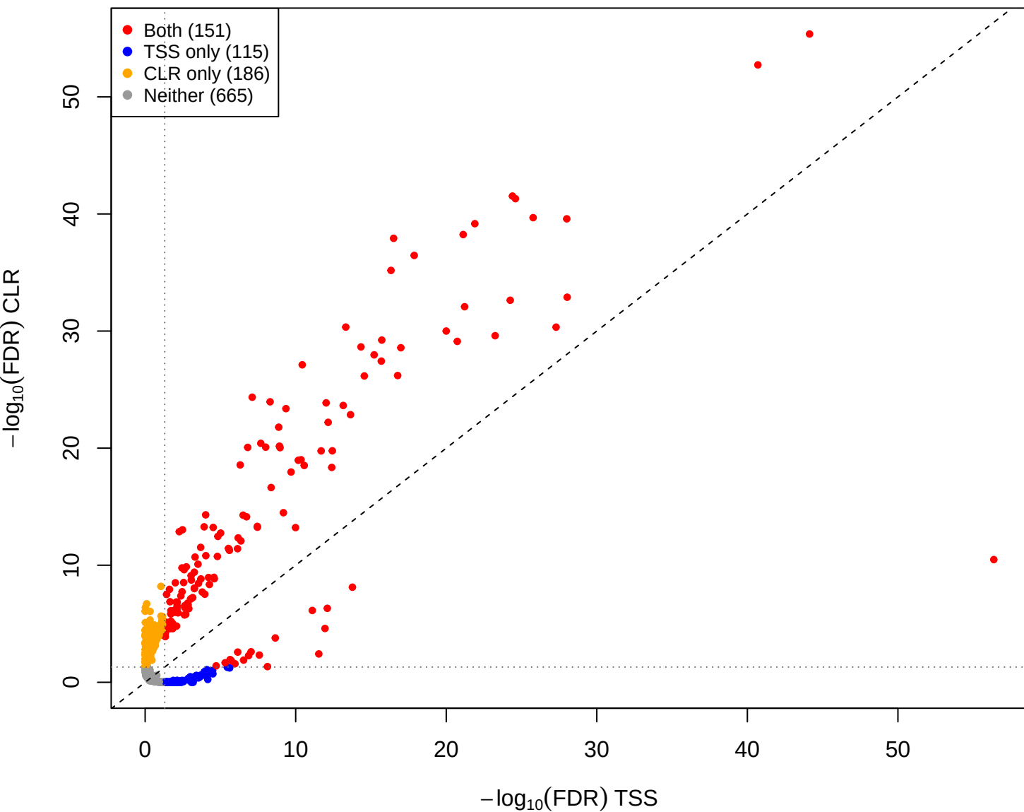
cent vs mid – CLR(const=1) vs TSS (gamma = 1e-05)
