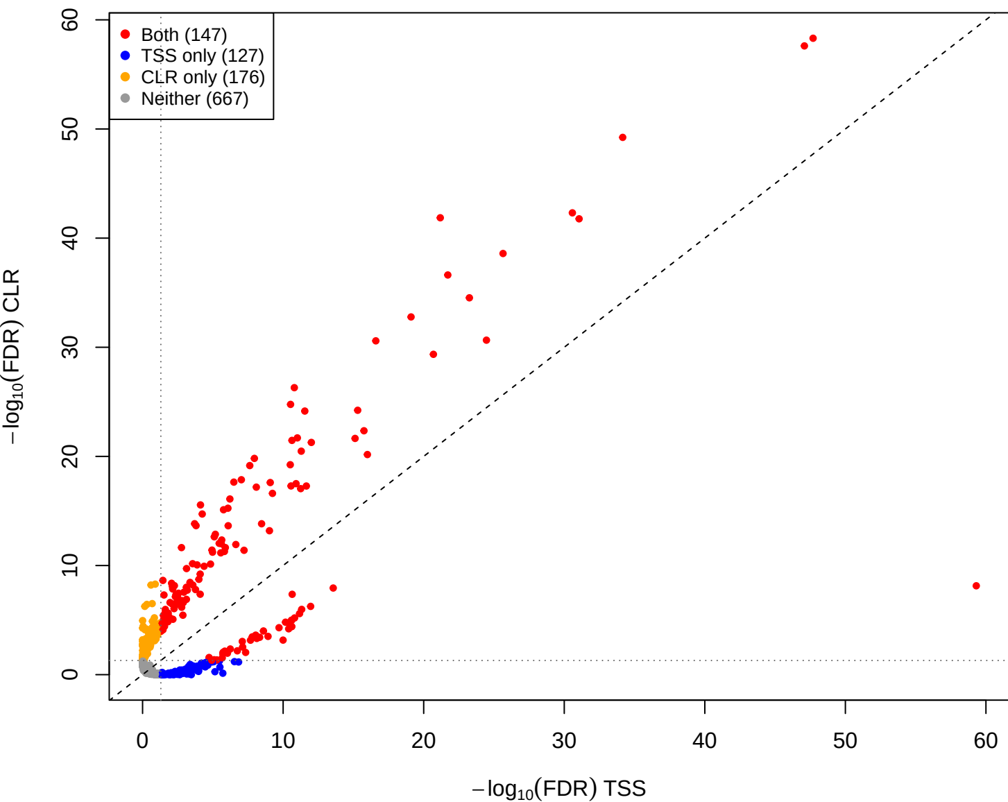
cent vs kin - CLR(const=1) vs TSS (gamma = 1e-05)
