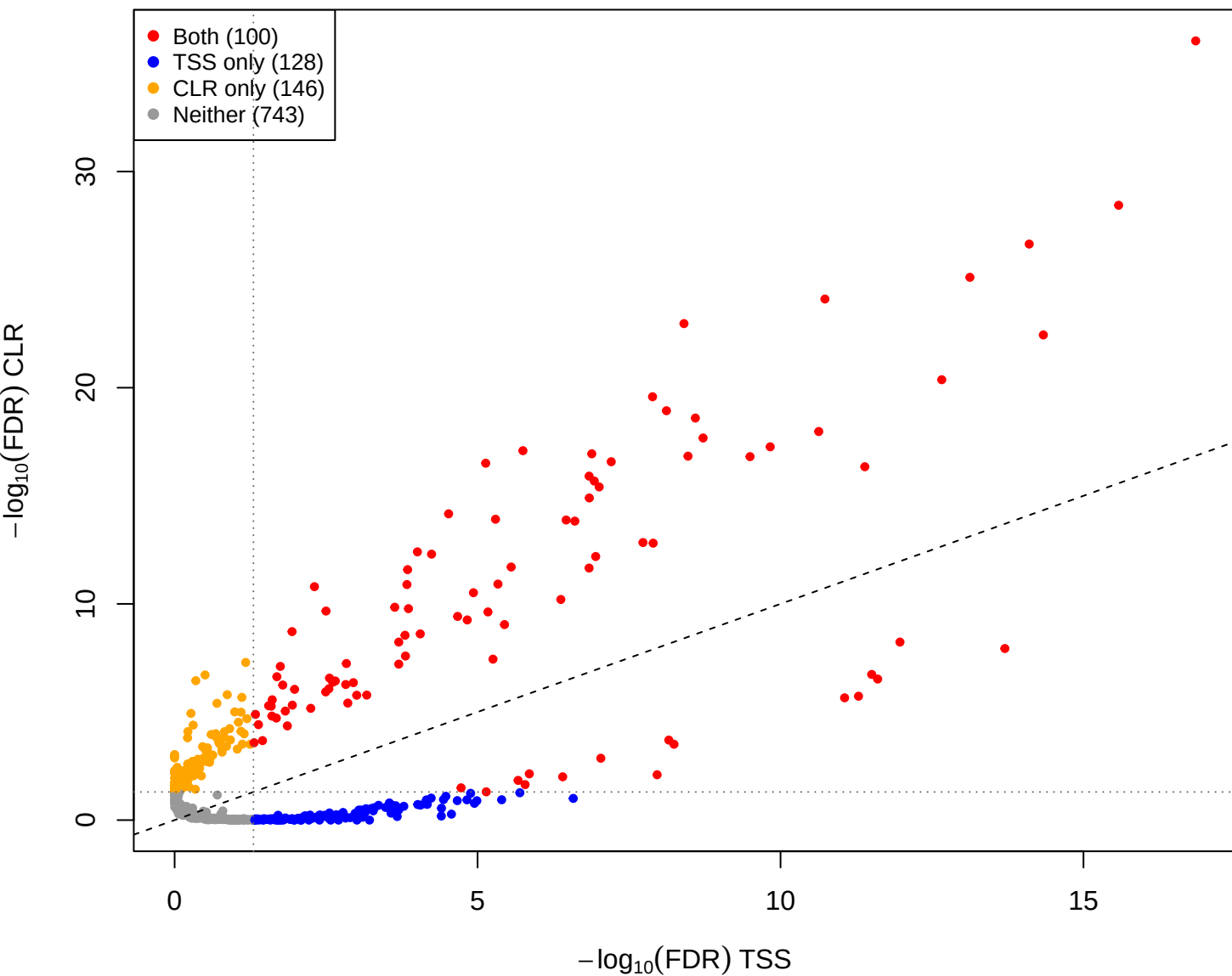
cent vs mage – CLR(const=1) vs TSS (gamma = 1e-05)
