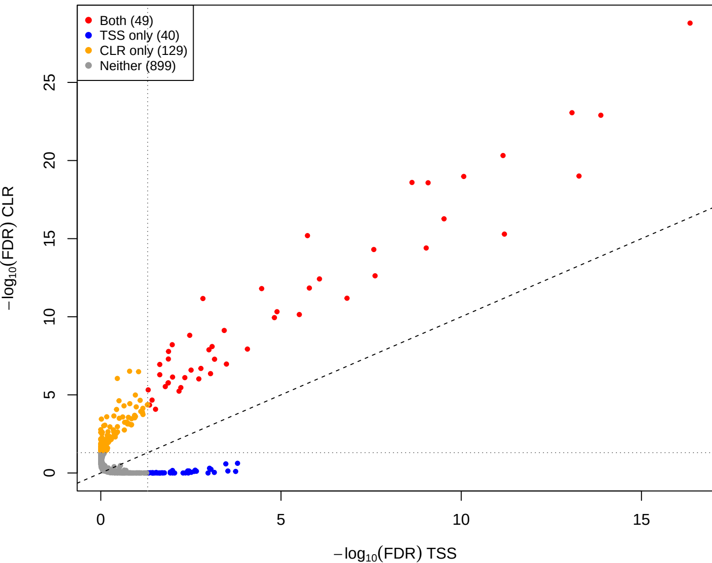
eld vs mage – CLR(const=1) vs TSS (gamma = 1e-05)
