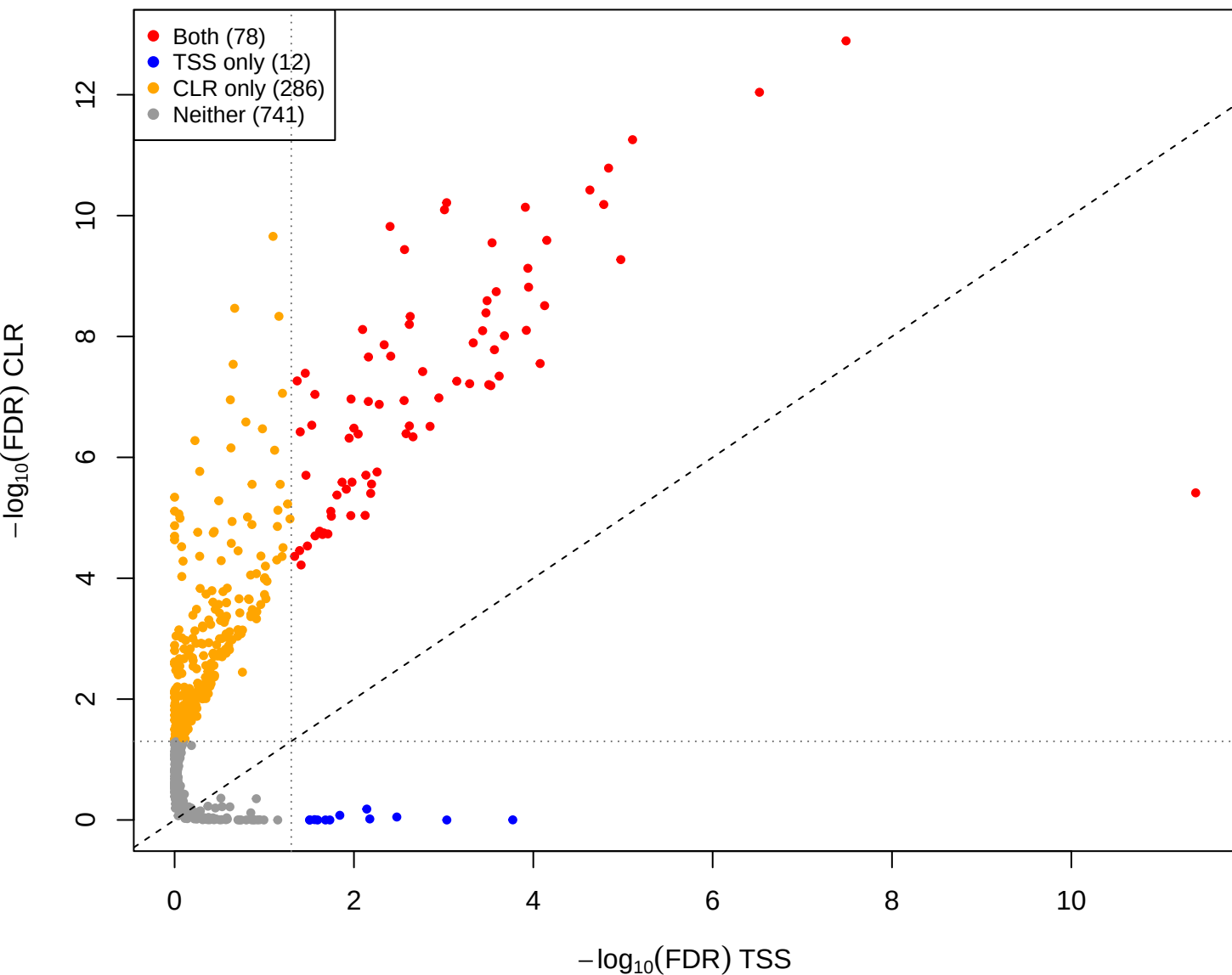
mage vs mid - CLR(const=1) vs TSS (gamma = 1e-05)
